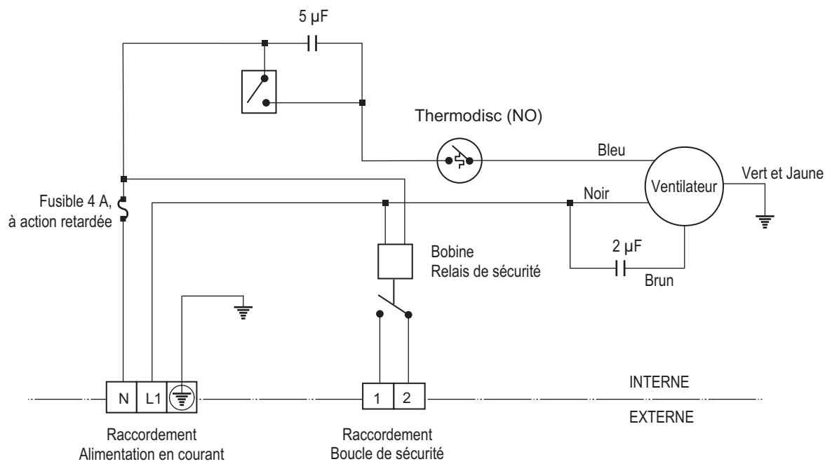
Figure 26 : Schéma de câblage Unité de ventilation Condair
