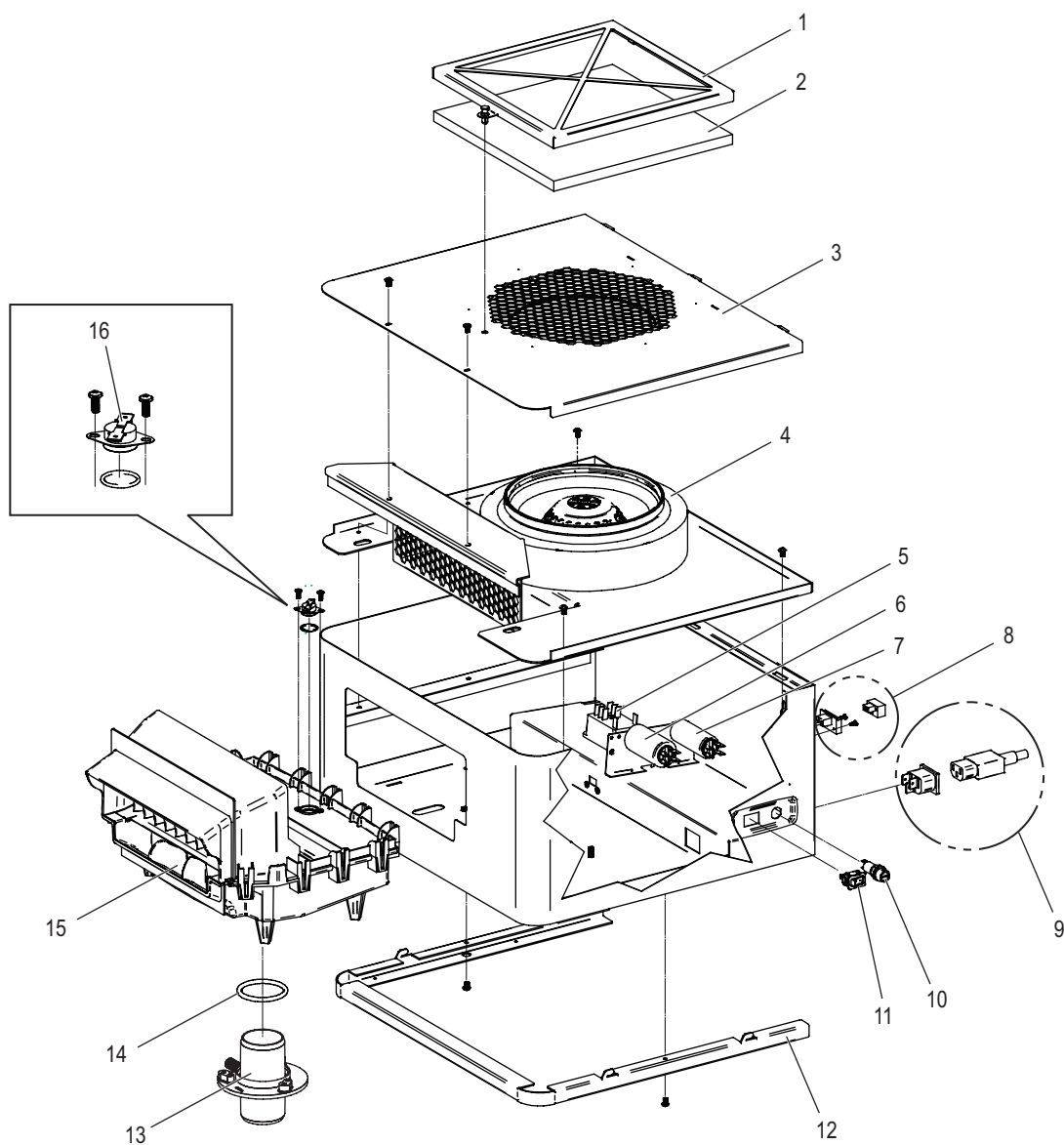
Figure 25 : Pièces de rechange Unité de ventilation Condair
