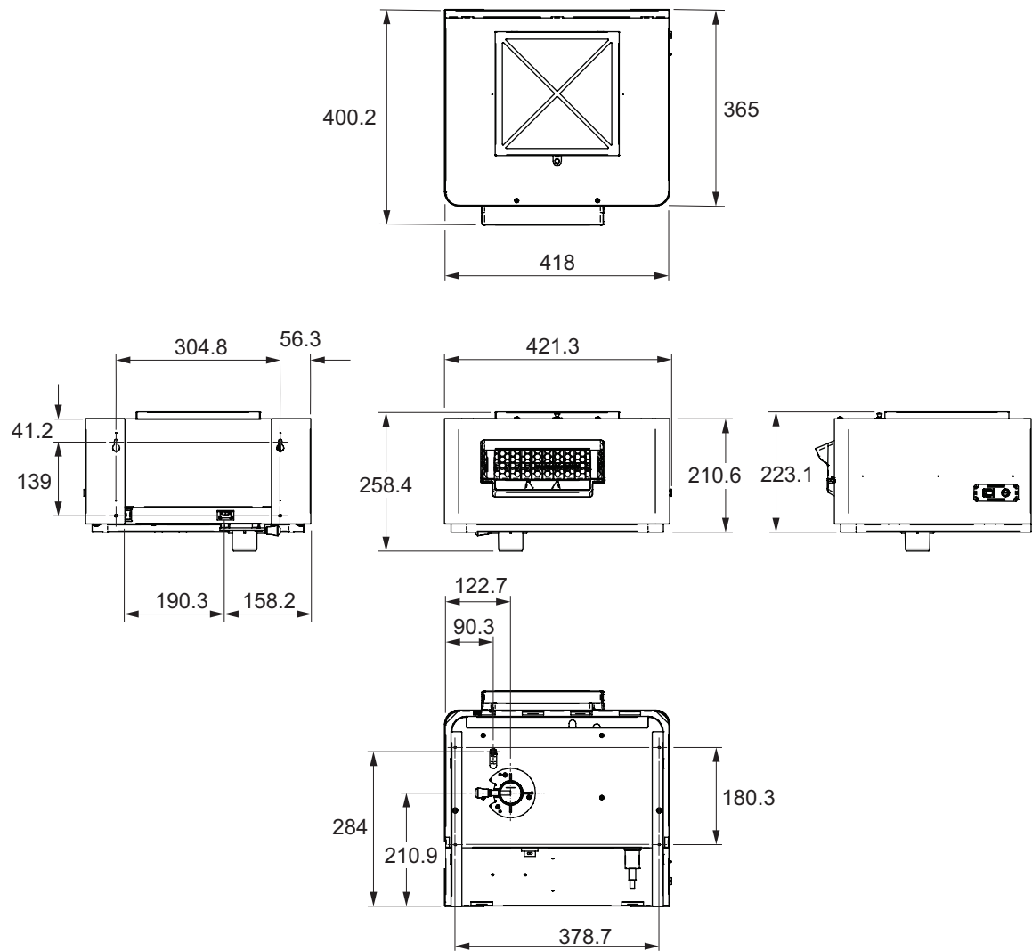
Figure 27 : Dimensions globales
