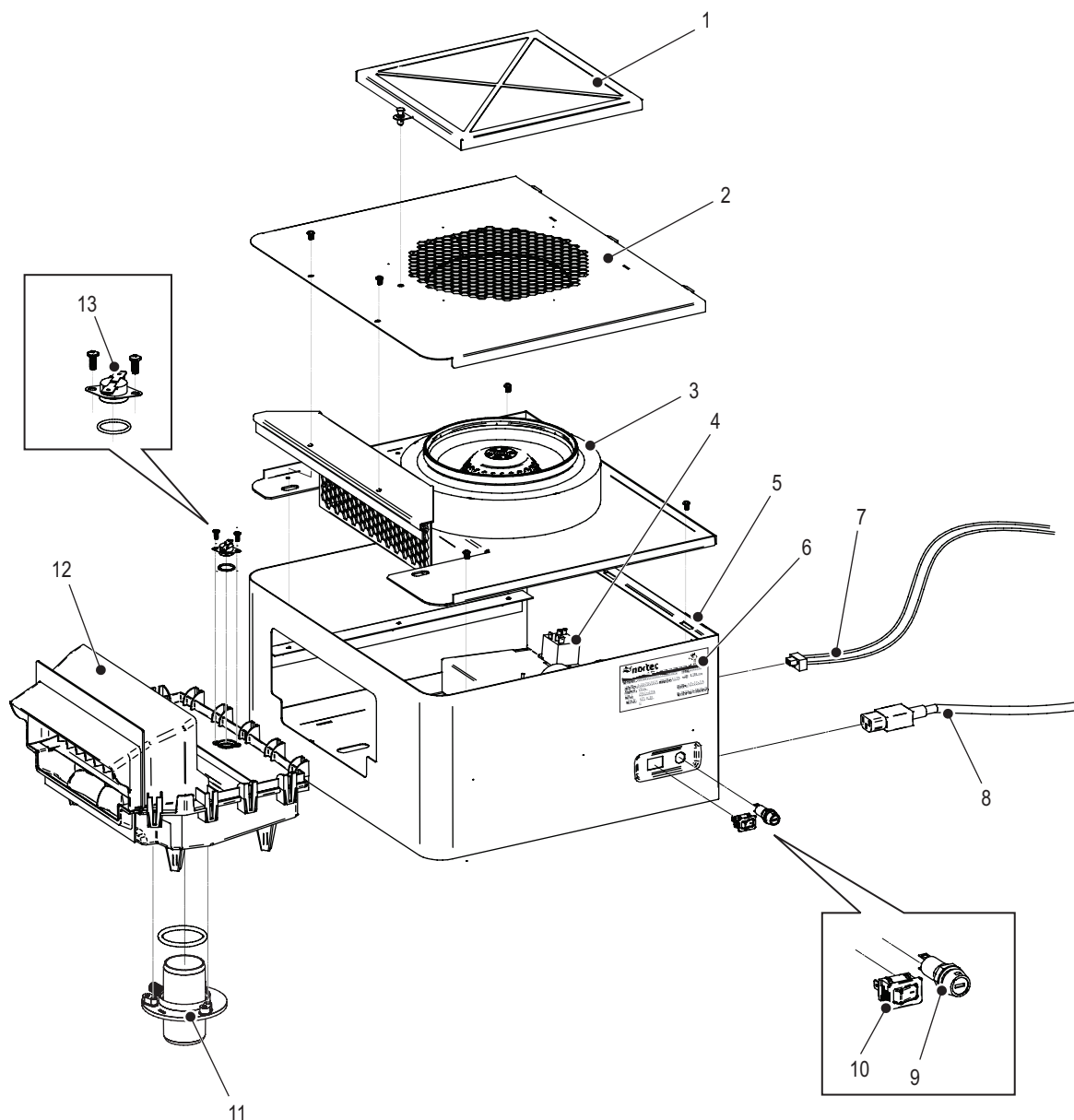
Figure 3 : Composants Unité de ventilation Condair
