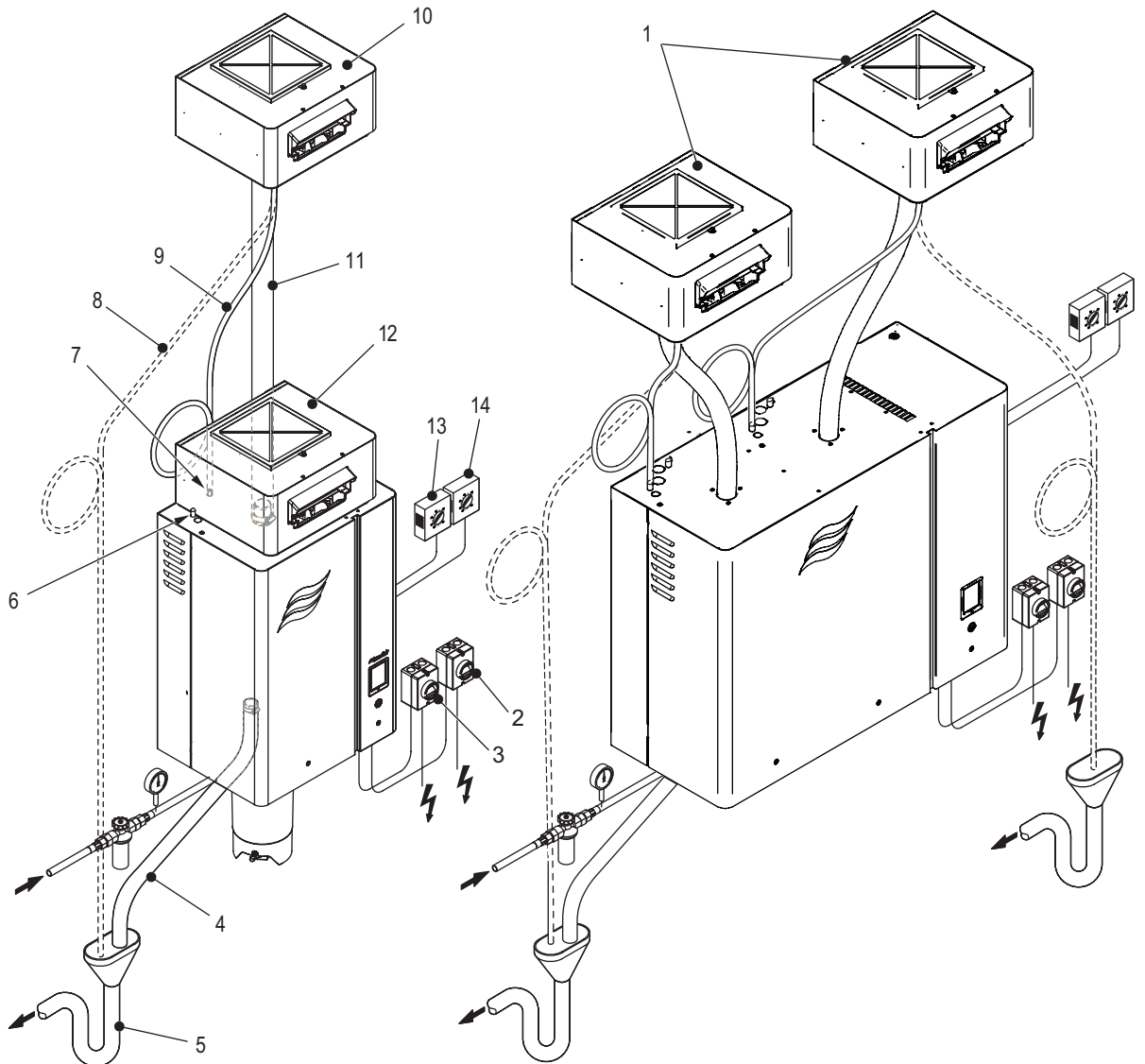
Figure 4 : Installation habituelle des unités de ventilation avec un humidificateur Condair EL/RS
