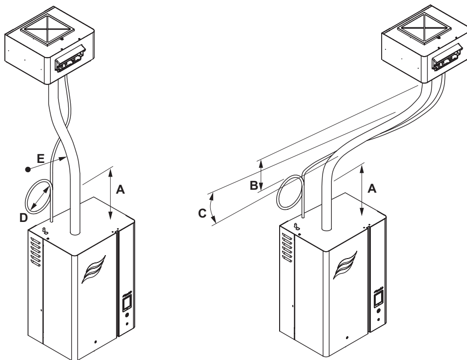
Figure 7 : Minima admissibles pour les conduites de vapeur et de condensat
