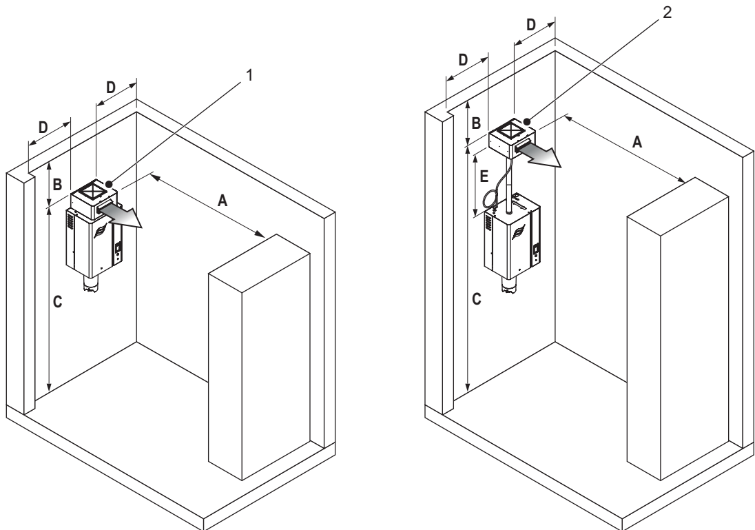
Figure 6 : Dégagements requis pour l'unité de ventilation
