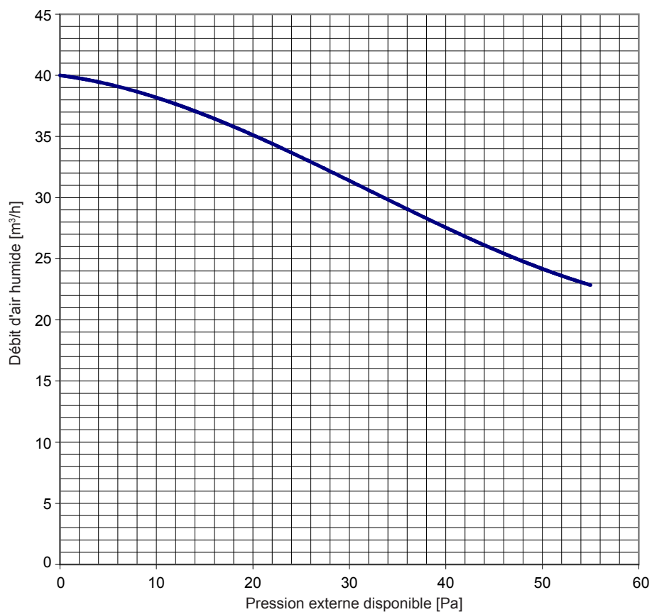
Fig. 9: Débit d'air humide Condair DA 210
