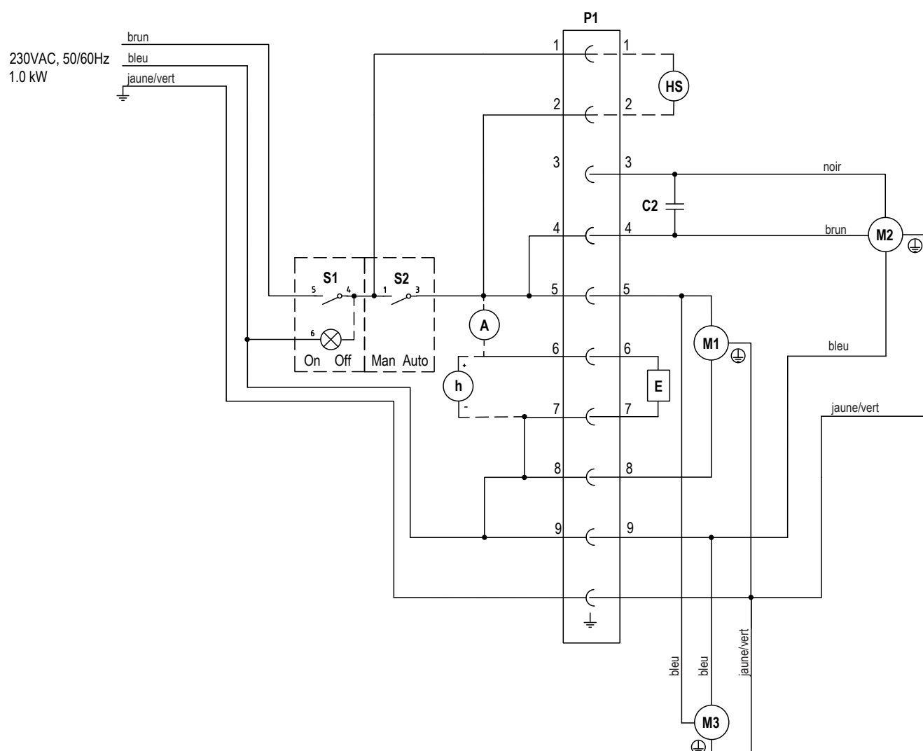
Fig. 12: Schéma du circuit électrique Condair DA 210
