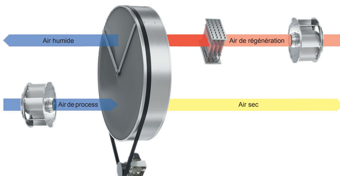
Fig. 2: Principe de fonctionnement DA 210
