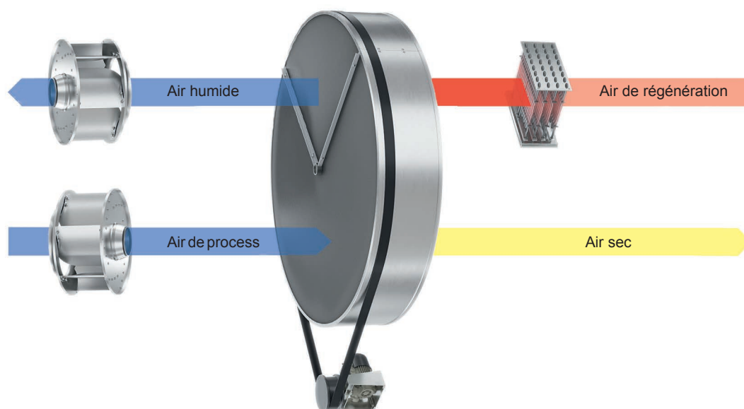
Fig. 3: Principe de fonctionnement DA 400 / DA 450
