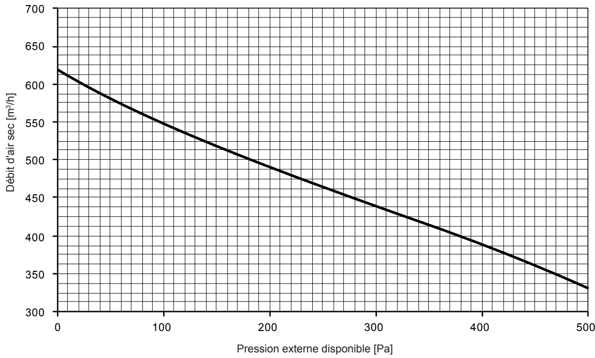
Fig. 10: Débit d'air sec Condair DA 400 / DA 450
