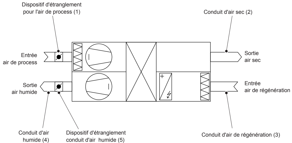
Fig. 5: Schéma d'installation DA 400 / DA 450
