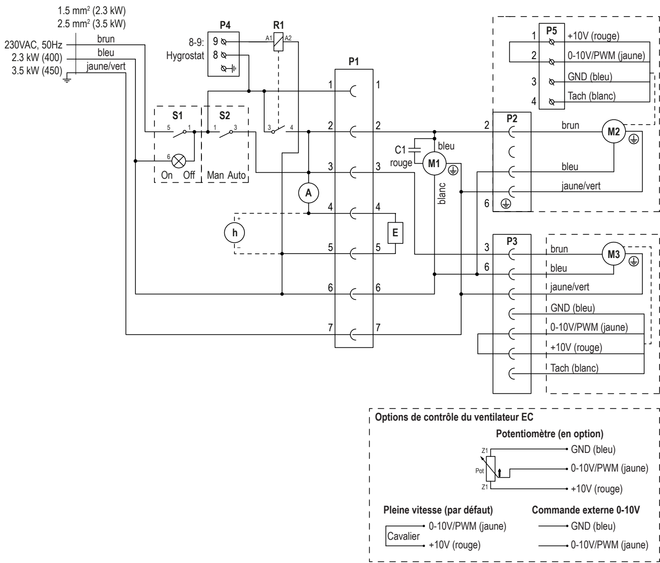
Fig. 13: Schéma du circuit électrique Condair DA 400 / DA 450
