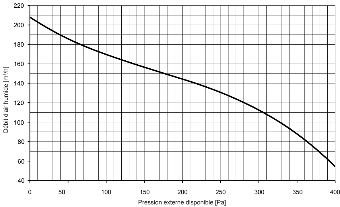
Fig. 11: Débit d'air humide Condair DA 400 / DA 450
