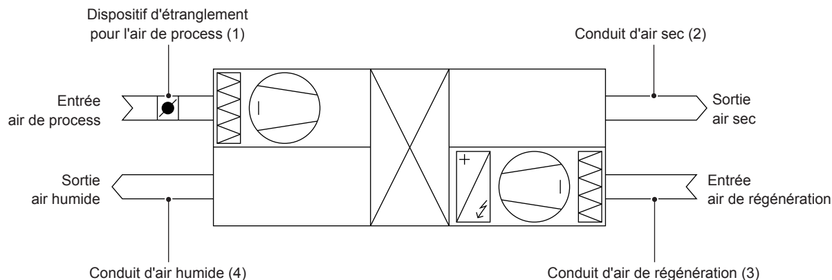
Fig. 4: Schéma d'installation DA 210
