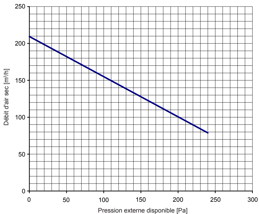
Fig. 8: Débit d'air sec Condair DA 210
