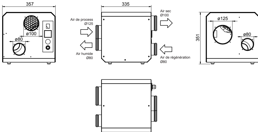
Fig. 6: Dimensions Condair DA 210 (en mm)
