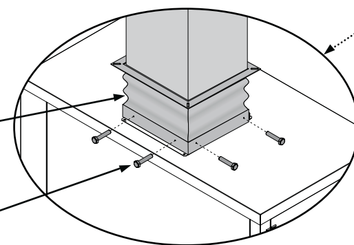
ASVE Soufflage vertical (version standard)
