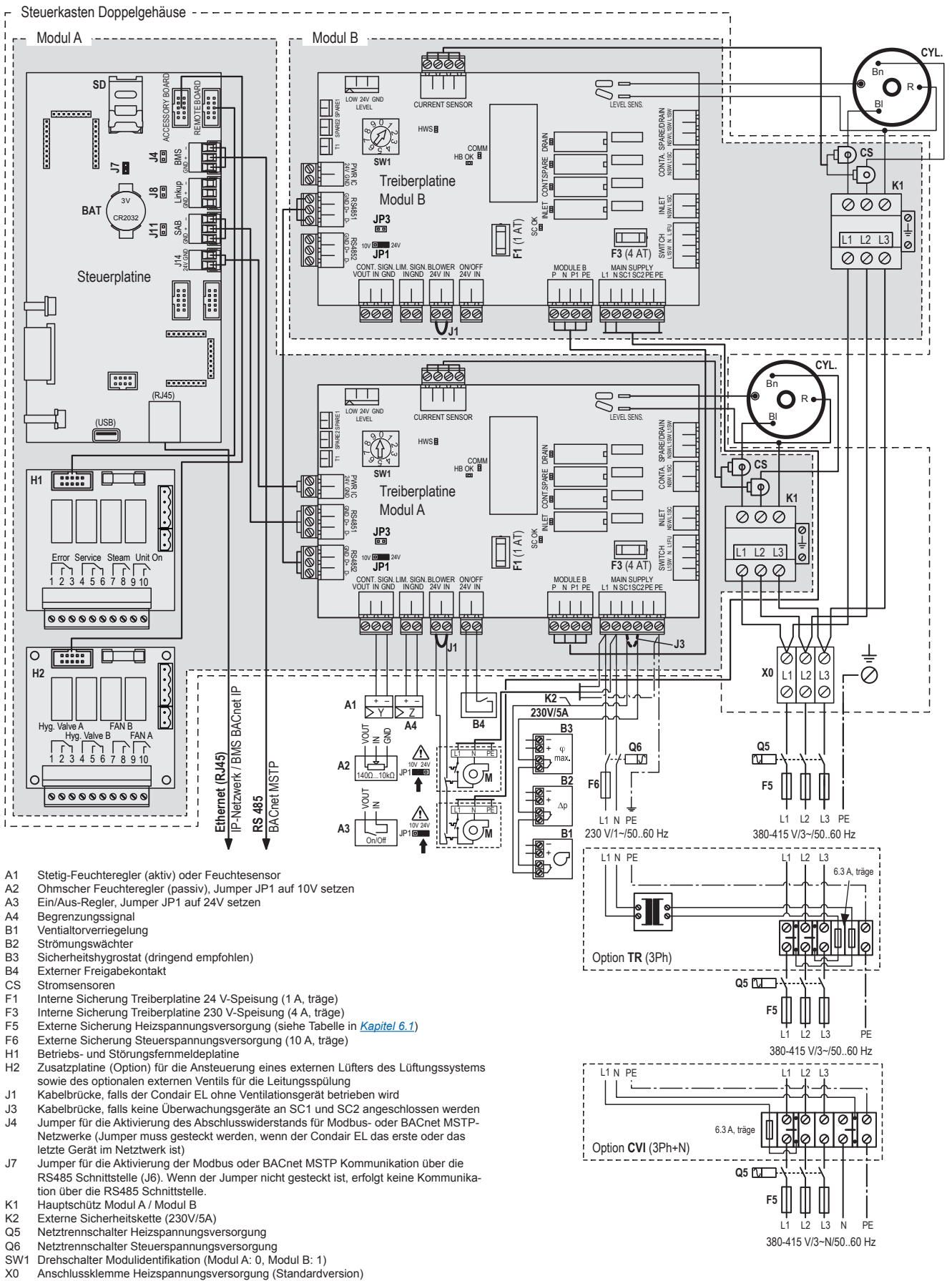
Abb. 25: Elektroschema Condair EL 50...90 - Einzelgeräte Gross ("L")
