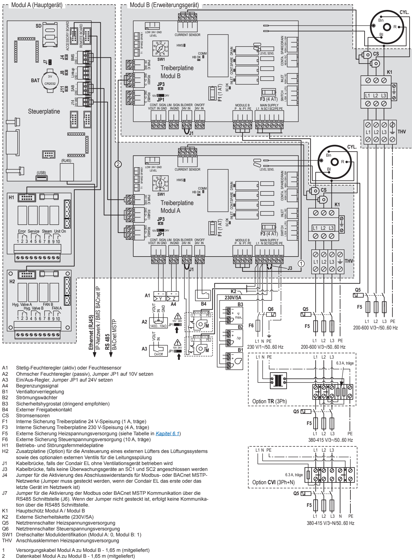
Abb. 26: Elektroschema Condair EL - Doppelgeräte (2 x "M") 35...90 kg/h
