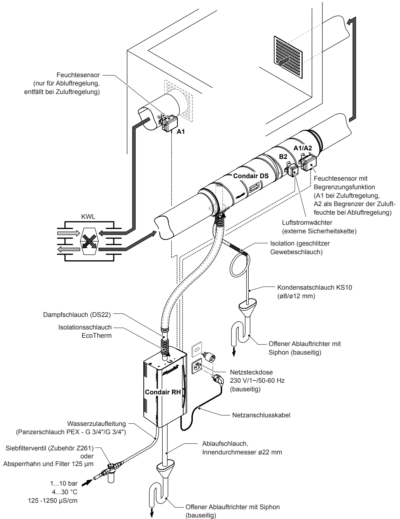
Abb. 3: Systemübersicht Condair RH mit Condair DS (Beispiel)
