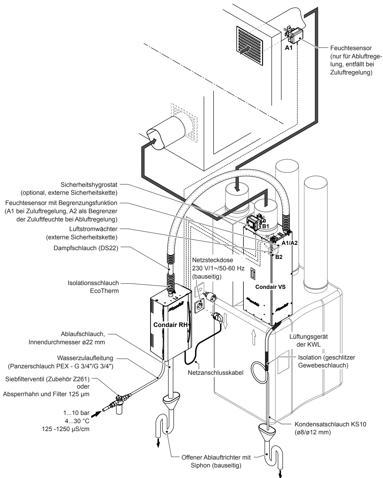
Abb. 2: Systemübersicht Condair RH mit Condair VS (Beispiel)
