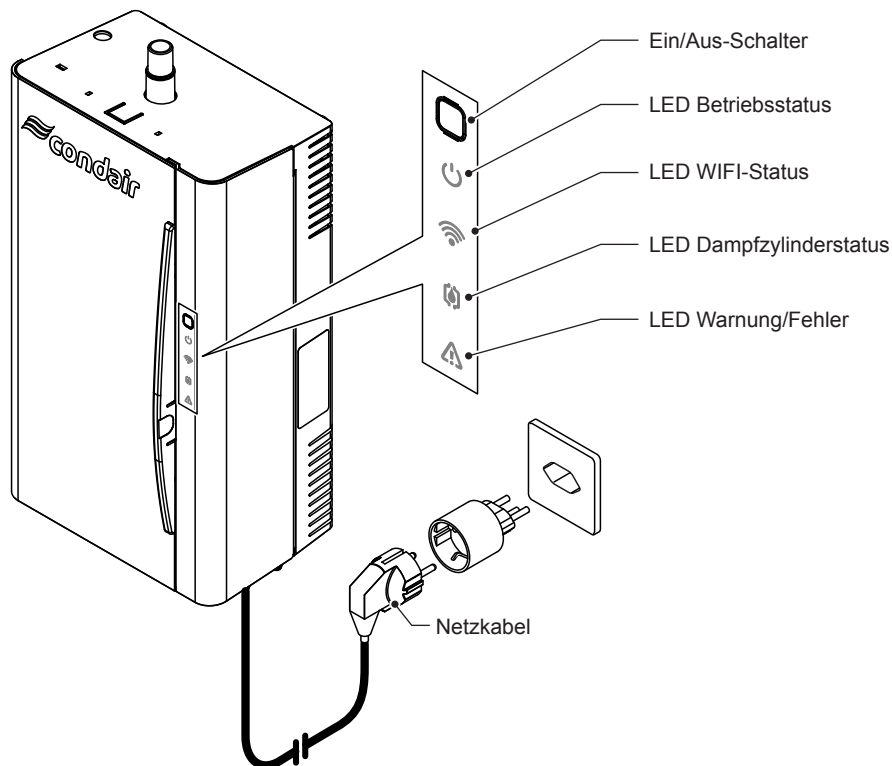
Abb. 9: Übersicht Anzeige- und Bedienelemente
