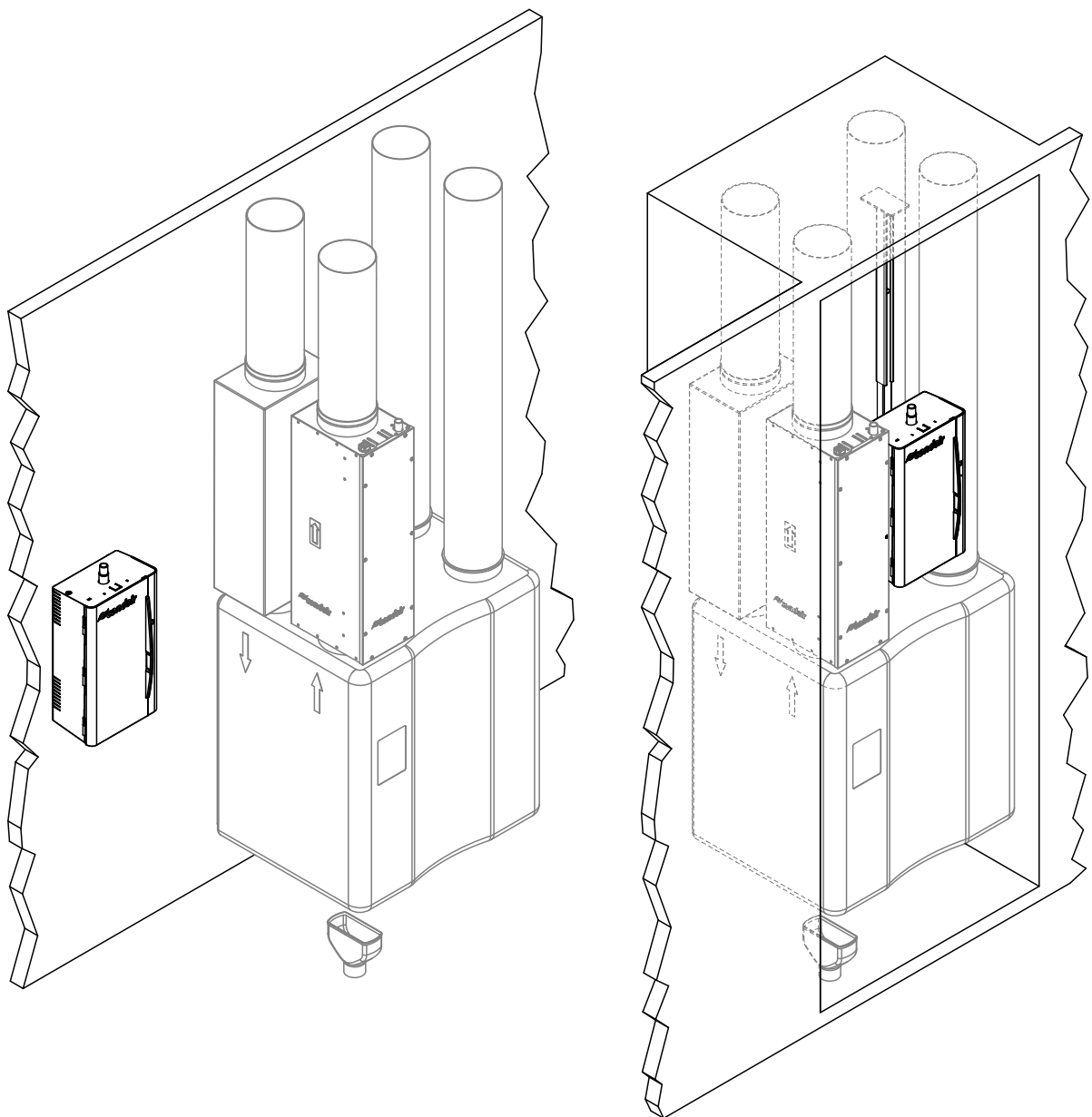
Abb. 6: Beispiel: Wand- und Deckenmontage Condair RH
