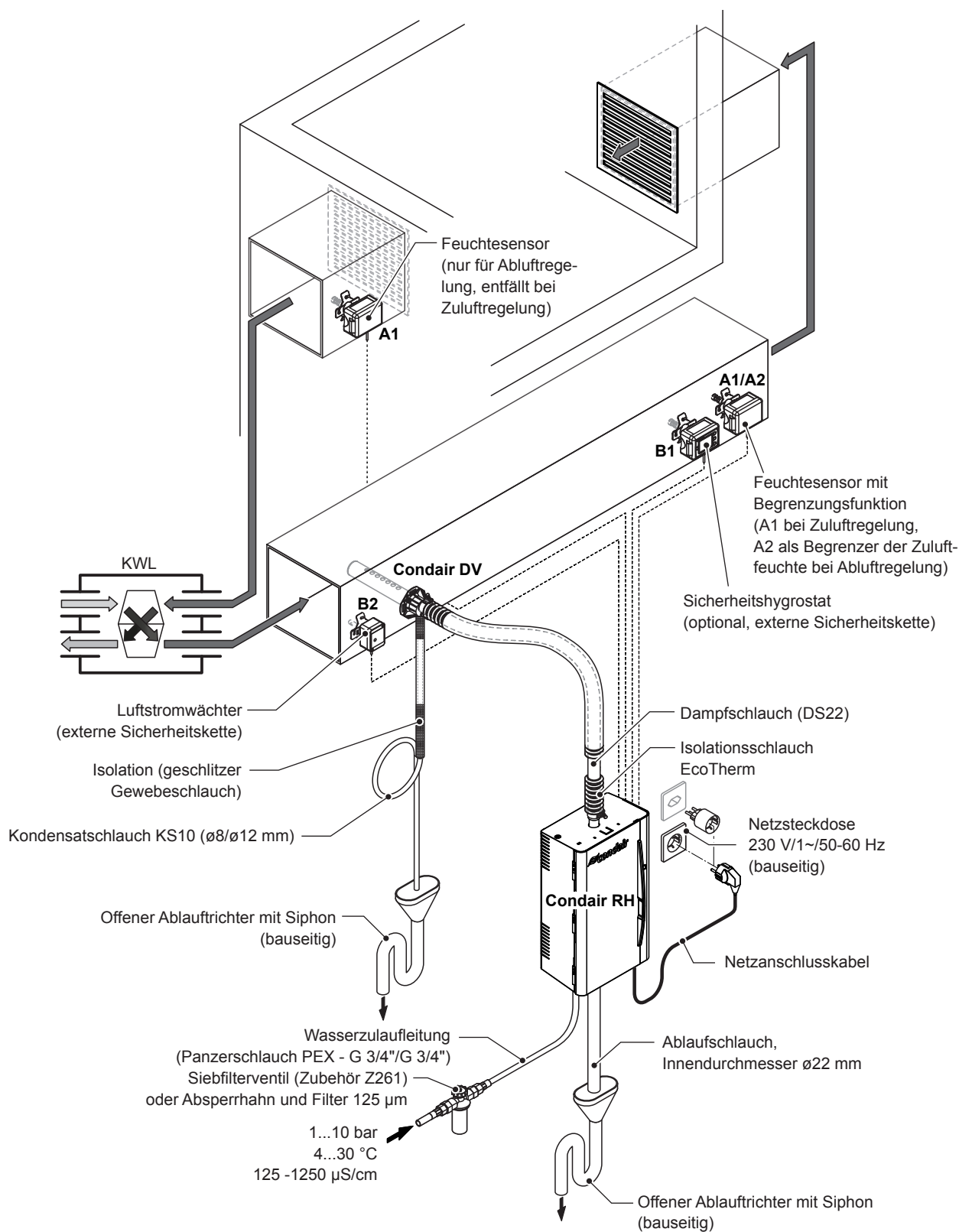
Abb. 4: Systemübersicht Condair RH mit Condair DV (Beispiel)
