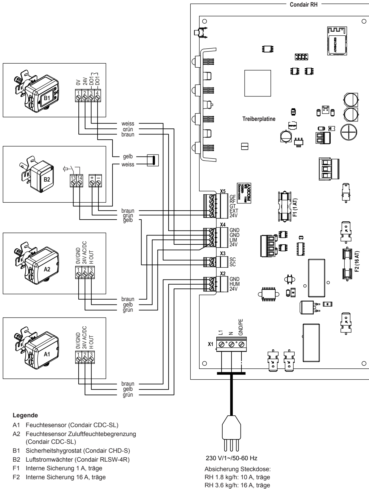
Abb. 8: Elektroschema Condair RH
