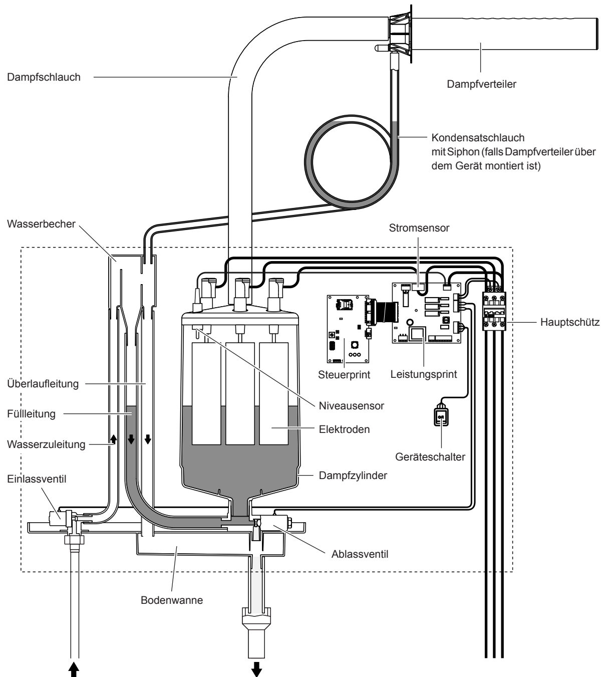
Abb. 3: Funktionsschema
