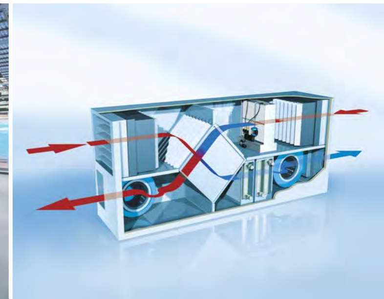
Refroidissement indirect par évaporation avec Condaire ME
