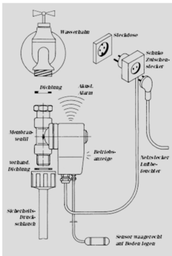
Wasserwächter mit Ventil 220–240 V 3/4" Sicherheitsdruckschlauch 3/4"
