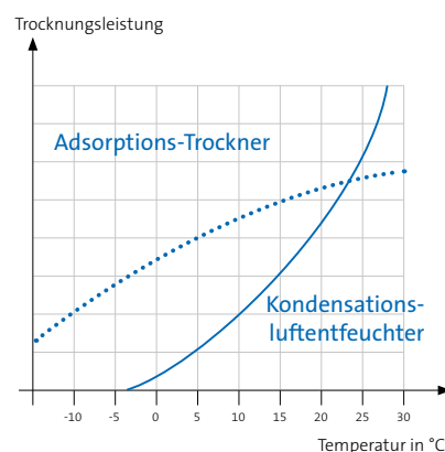
Leistungscharakteristik
