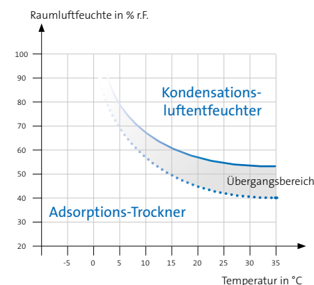
Empfohlener Einsatzbereich nach Temperatur/Feuchte
