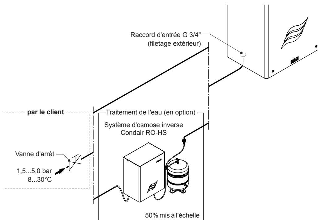
Fig. 18: Alimentation d'eau propre
