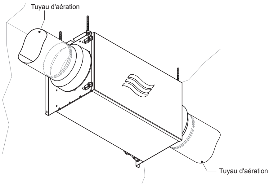
Fig. 10: Monter les tuyaux d'aération
