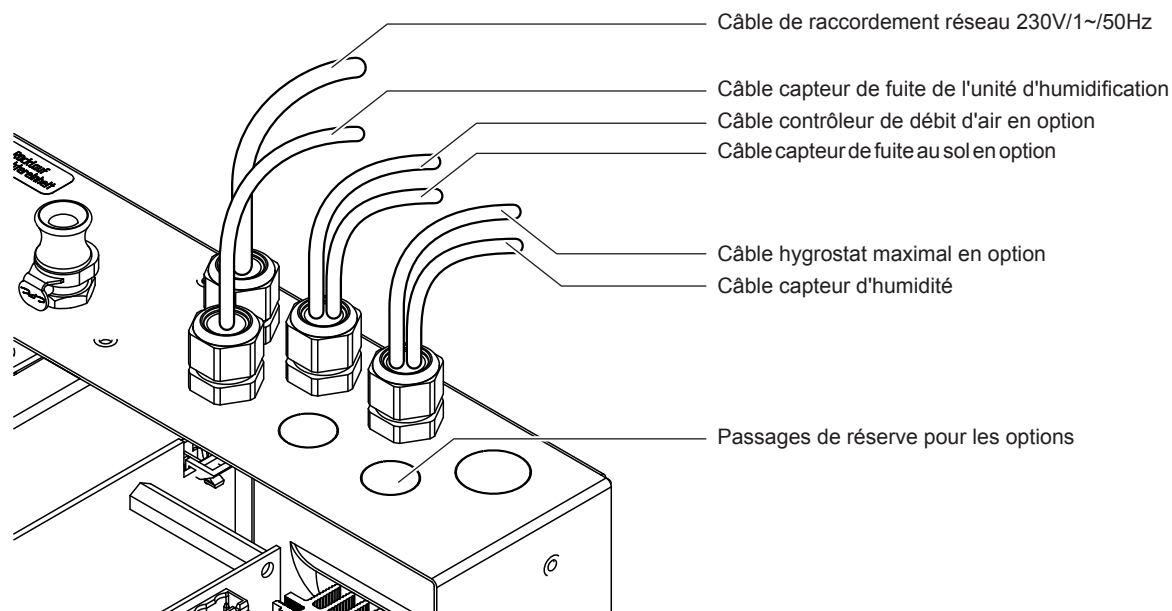
Fig. 26: Entrée des câbles
