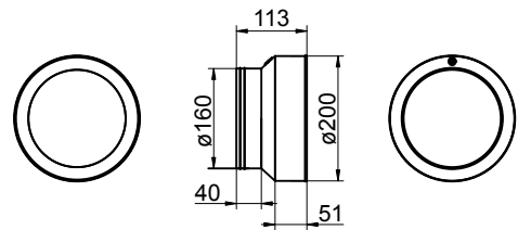
Fig. 29: Dimensions de raccord de transition DN160 (dimensions en mm)
