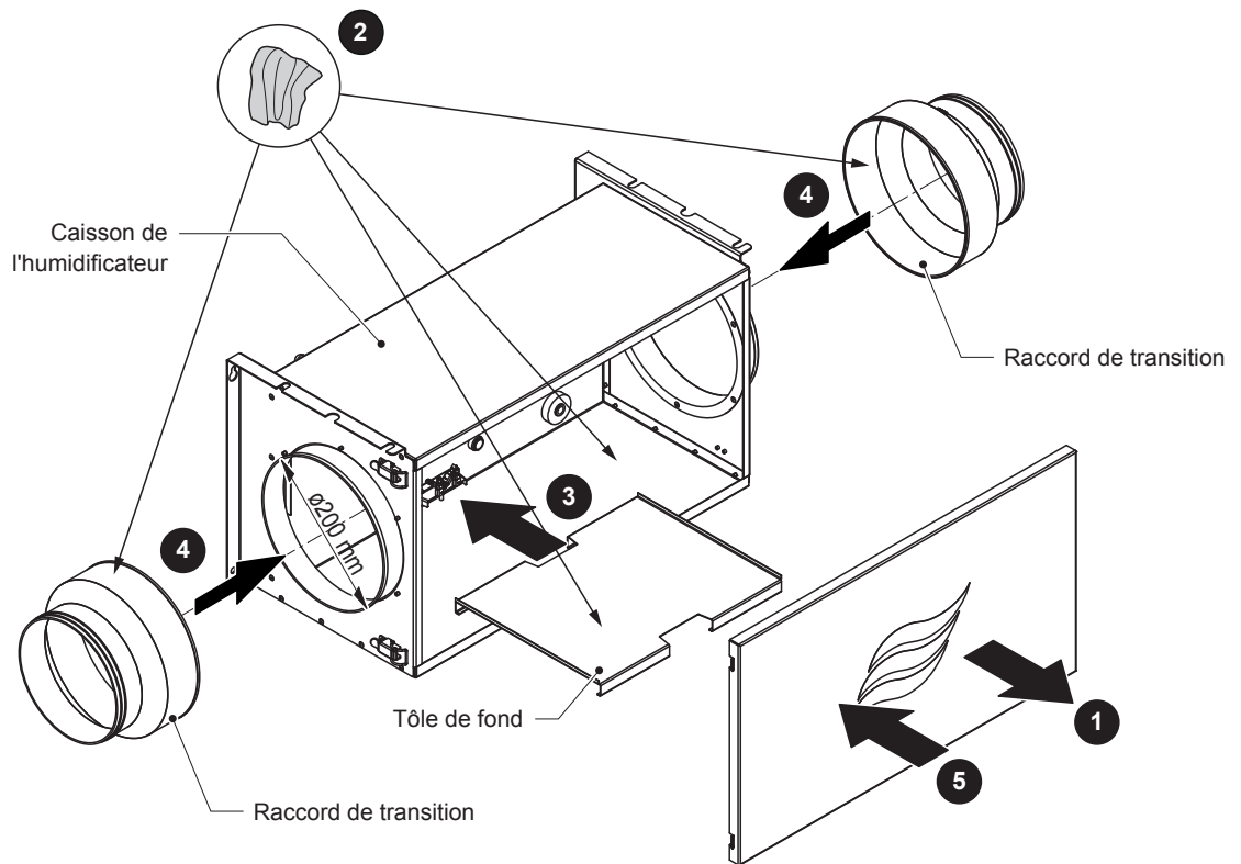
Fig. 6: Insérer la tôle de fond et installer les raccords de transition
