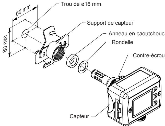
Fig. 23: Montage du capteur d'humidité et de température et de l'hygrostat maximal
