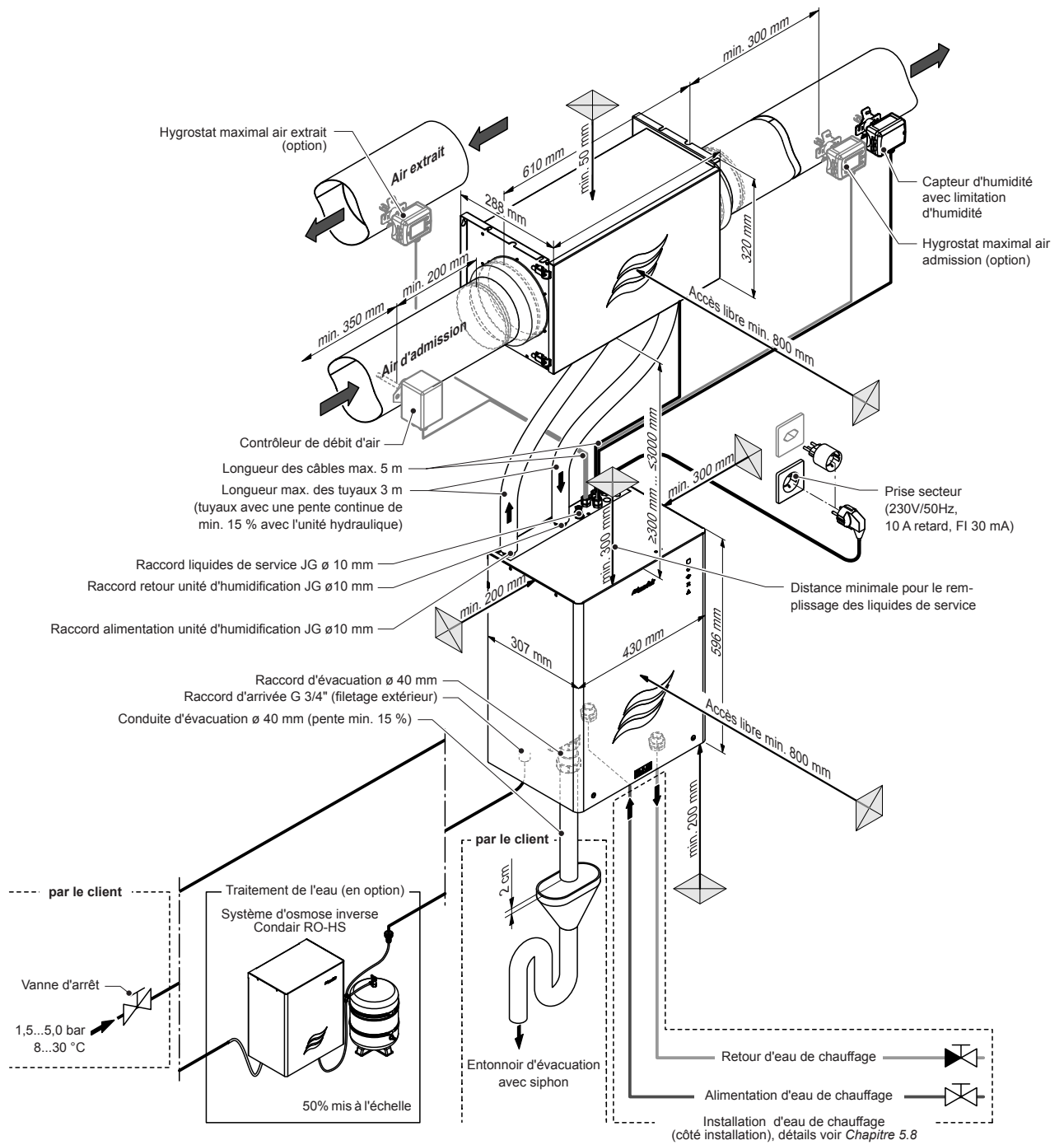
Fig. 2: Aperçu de l'installation du Condair MD, variante MD-EL-H
