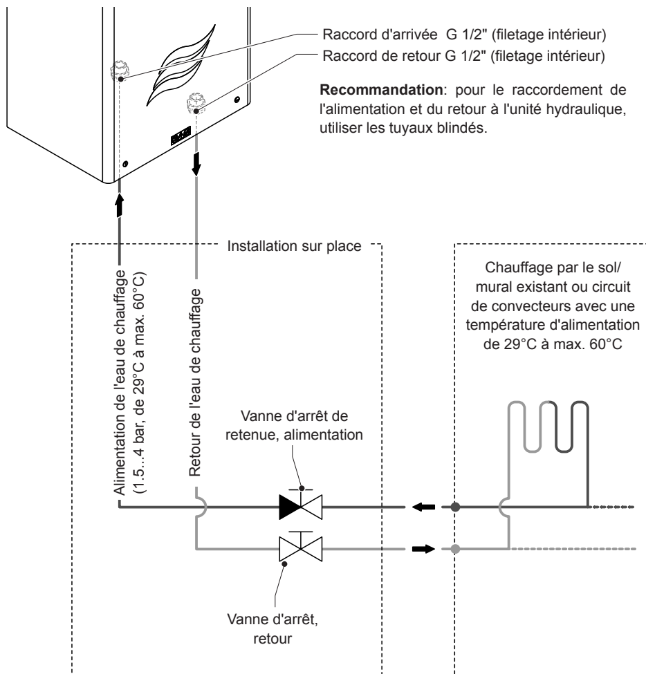
Fig. 20: Vue d'ensemble de l'installation raccordement eau de chauffage
