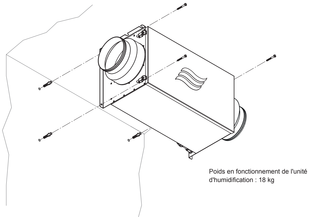
Fig. 14: Fixer le caisson de l'humidificateur au mur
