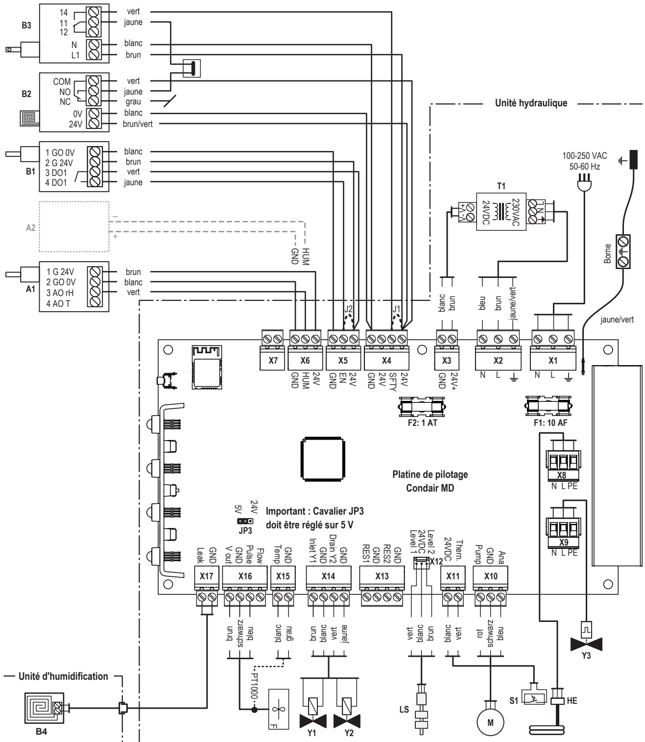
Fig. 25: Schéma électrique Condair MD
