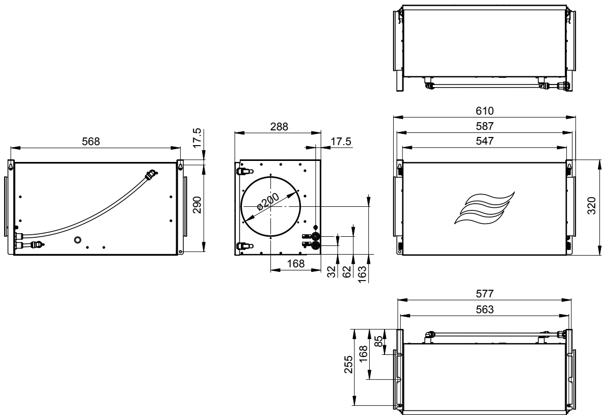
Fig. 27: Dimensions unité d'humidification (dimensions en mm)
