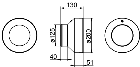
Fig. 28: Dimensions de raccord de transition DN125 (dimensions en mm)
