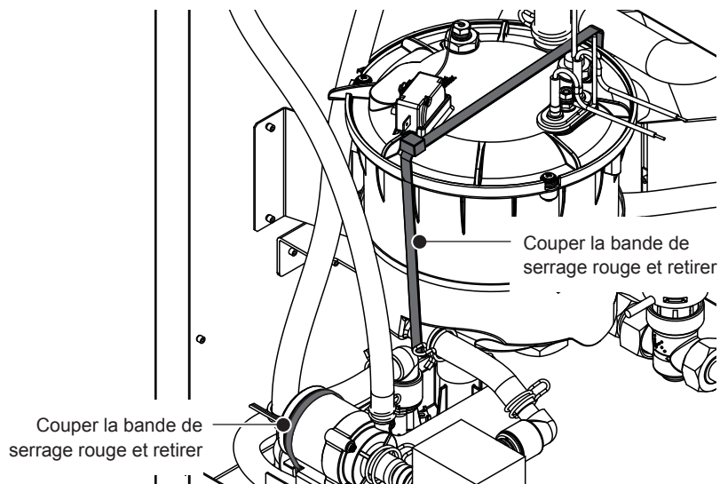
Fig. 16: Retirer les bandes de serrages rouges (sécurité de transport)
