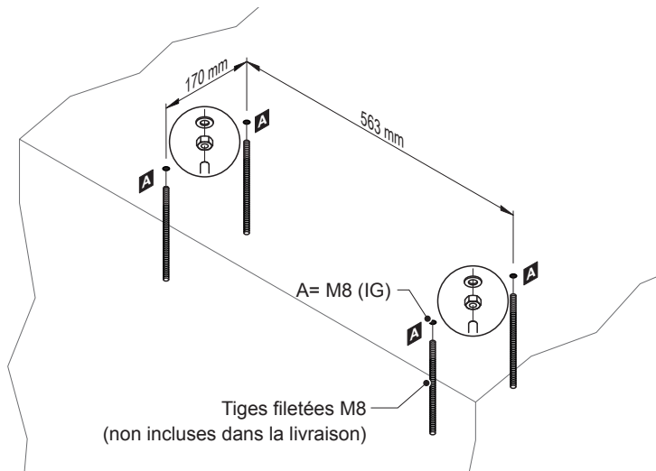
Fig. 7: Déterminer les points de fixation et monter les tiges filetées
