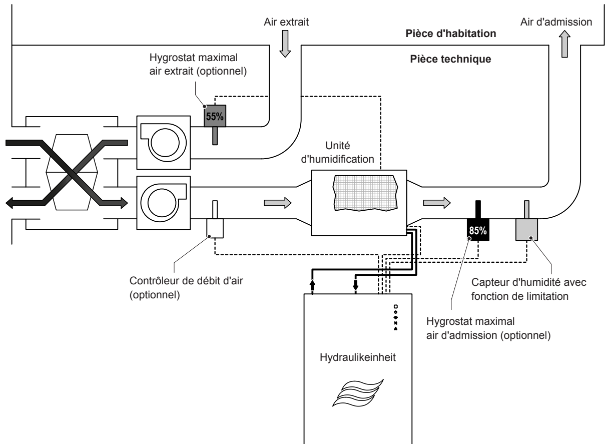
Fig. 21: Schéma de base de la régulation de l'humidité de l'air d'admission
