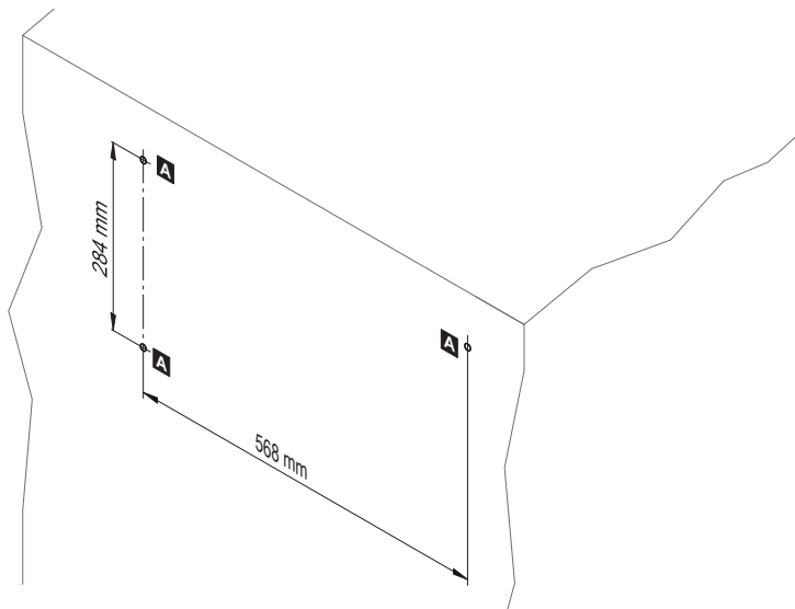
Fig. 13: Définir les points de fixation
