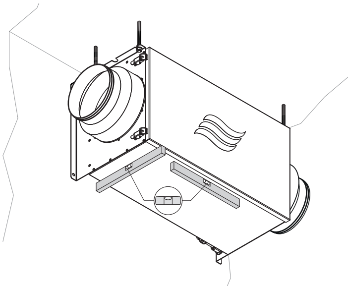
Fig. 9: Ajuster le caisson de l'humidificateur et serrer les raccords vissés
