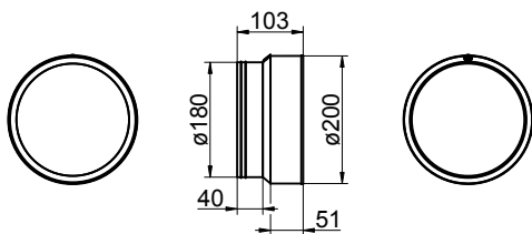
Fig. 30: Dimensions de raccord de transition DN180 (dimensions en mm)
