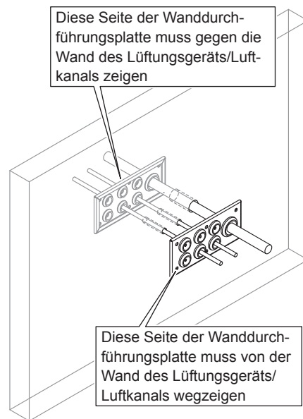
Abb. 27: Wanddurchführungsplatte montieren (Innenmontage)
