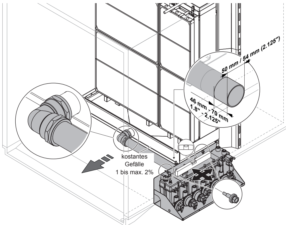
Abb. 20: Hydraulikmodul montieren (Aussenmontage, Wassertank mit Zentralablauf)
