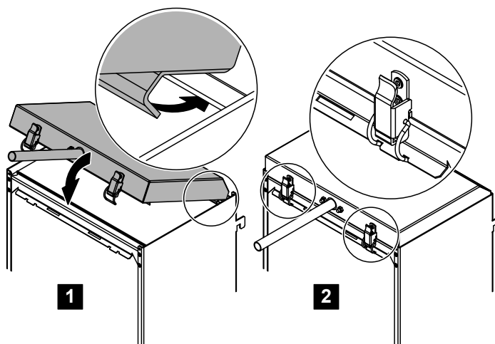
Abb. 13: Verteilhaube auf der obersten Polyester-Verdunsterkassette montieren
