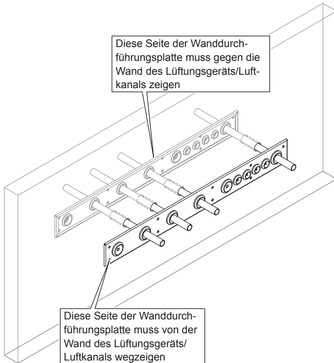
Abb. 26: Wanddurchführungsplatte montieren (Aussenmontage)
