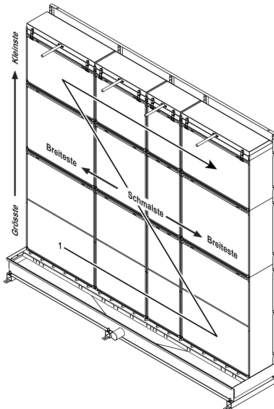
Abb. 15: Montagereihenfolge und Positionierung der Verdunsterkassetten
