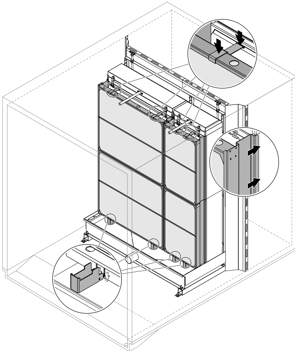
Abb. 17: Vertikale Reihen der Tropfenabscheiderkassetten montieren
