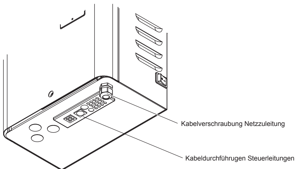
Abb. 34: Kabeldurchführungen an der Steuereinheit
