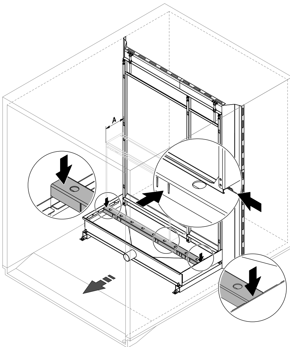
Abb. 11: Querträger montieren
