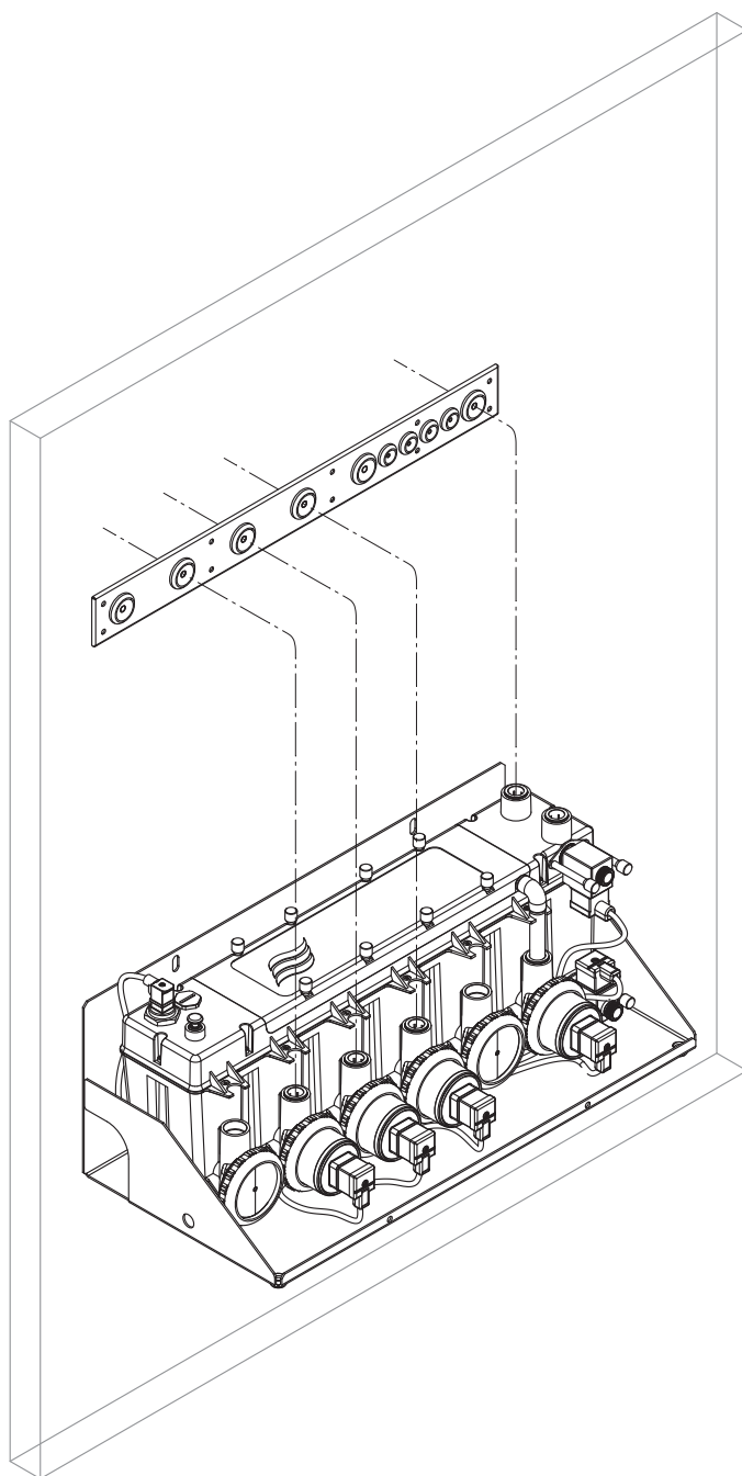
Abb. 22: Durchführungsbohrungen markieren (Aussenmontage)
