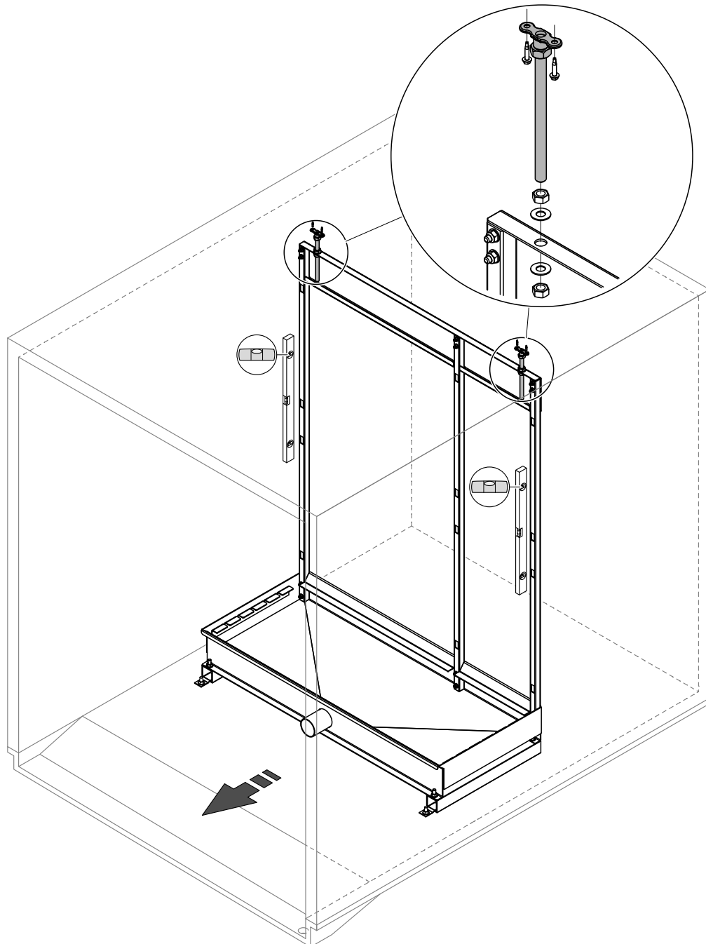
Abb. 8: Querstrebe an der Kanaldecke befestigen
