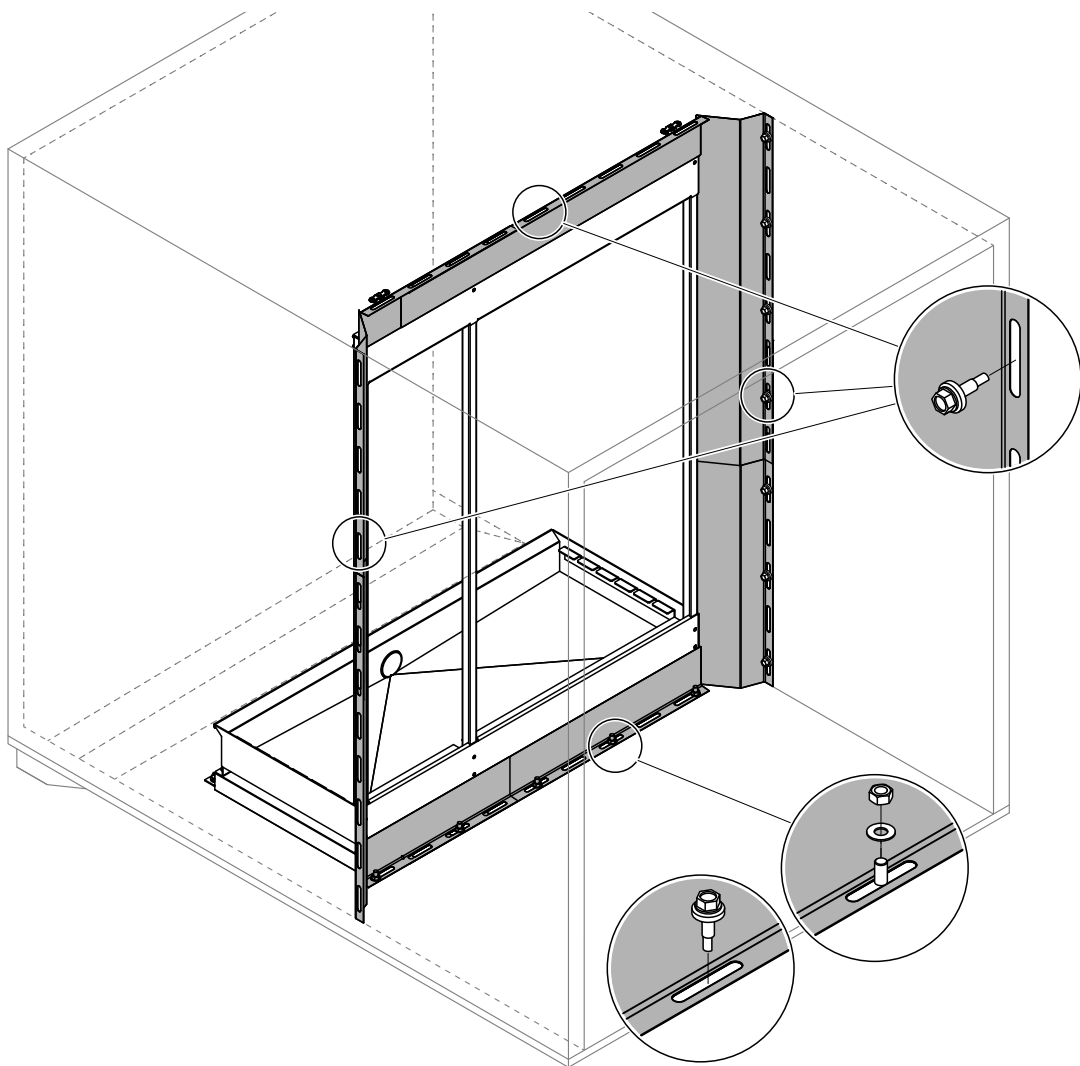
Abb. 9: Optionale Condair Abdichtbleche auf der Lufteintrittsseite montieren
