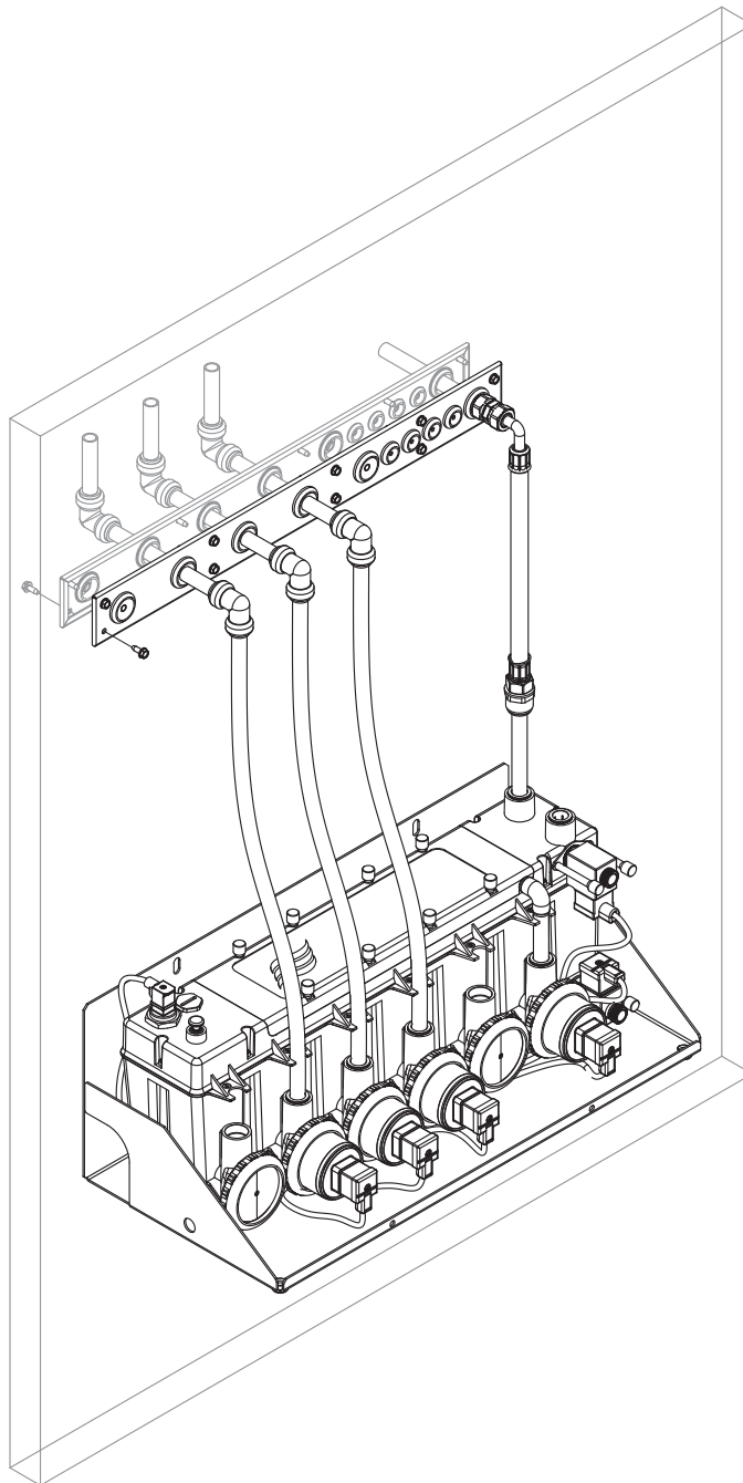
Abb. 28: Wanddurchführungsplatte an der Wand des Lüftungsgeräts/Luftkanals befestigen (Aussenmontage)
