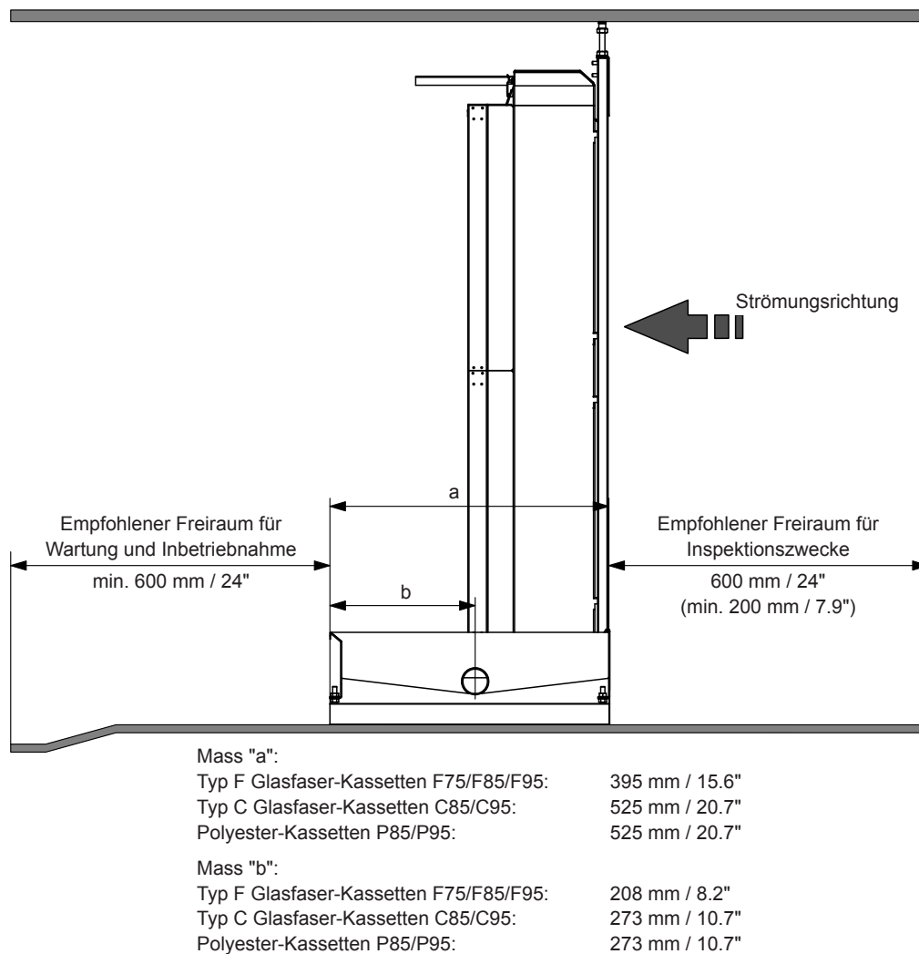
Abb. 4: Positionierung des Verdunstermoduls (Tank mit Seitenablauf)
