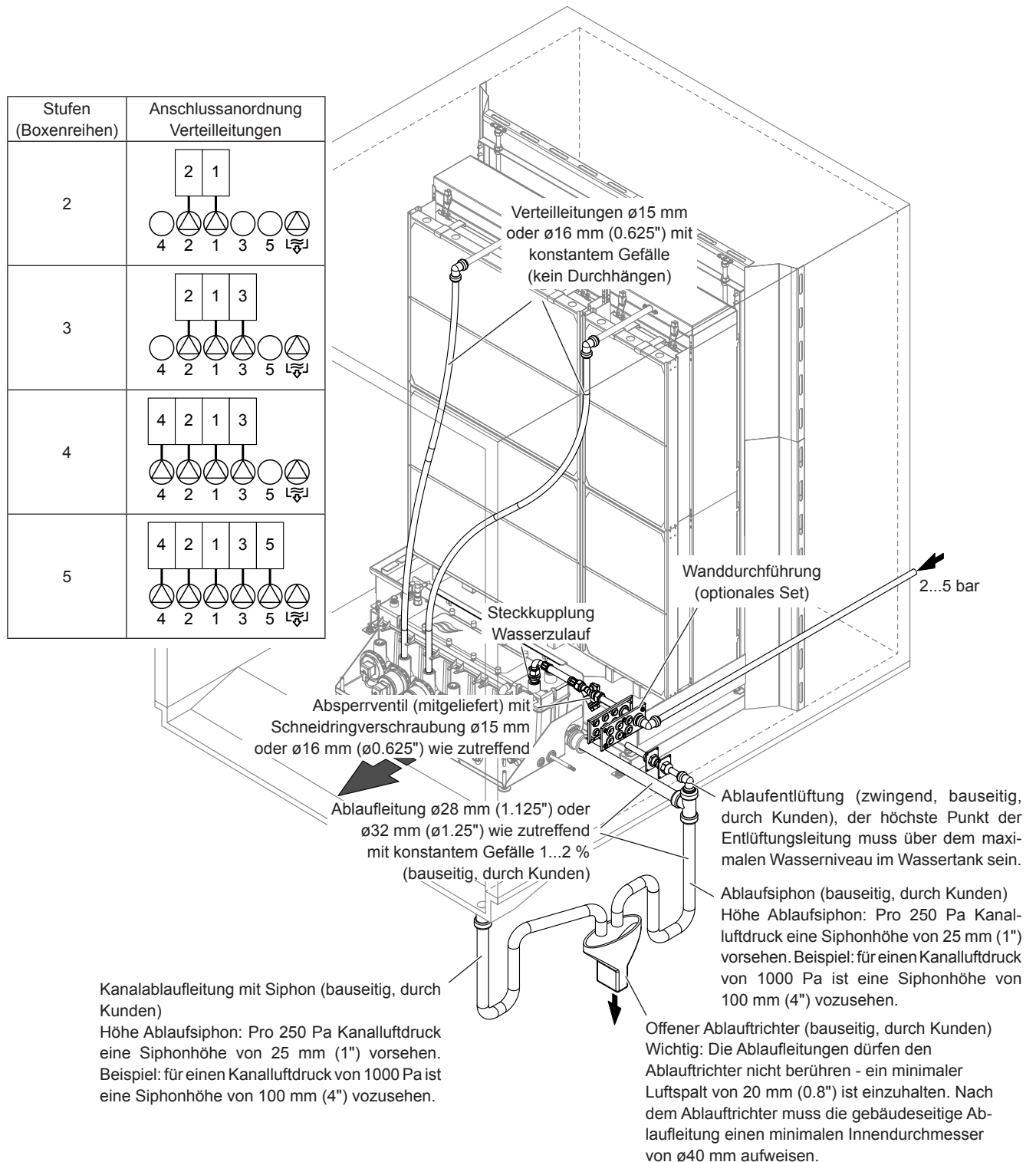
Abb. 30: Wasserinstallation (Innenmontage)
