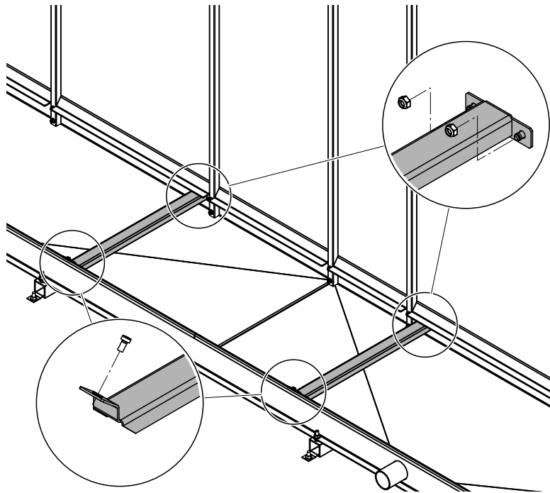
Abb. 10: Querträgerabstützung(en) montieren
