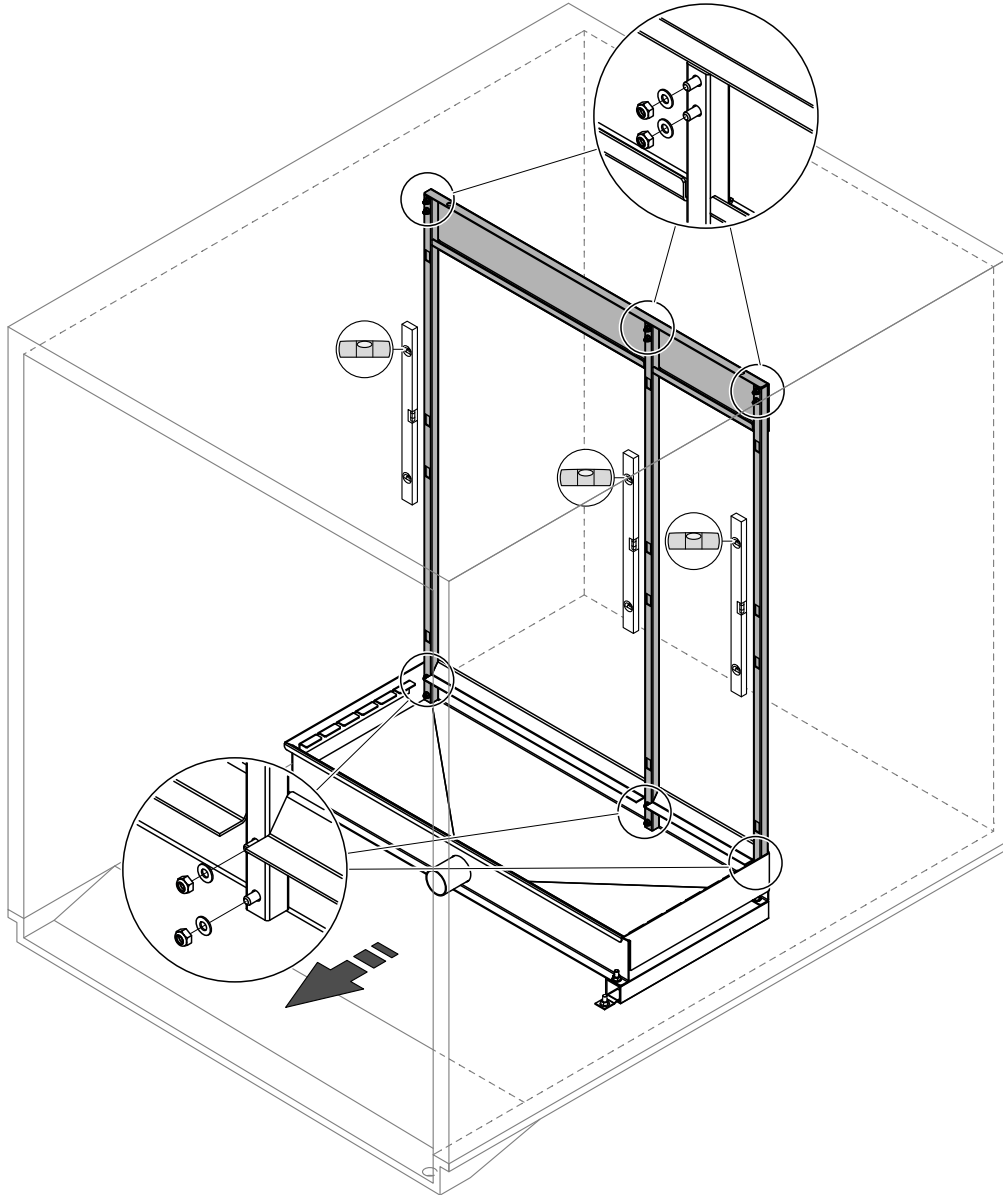
Abb. 7: Trägerrahmen am Wassertank befestigen
