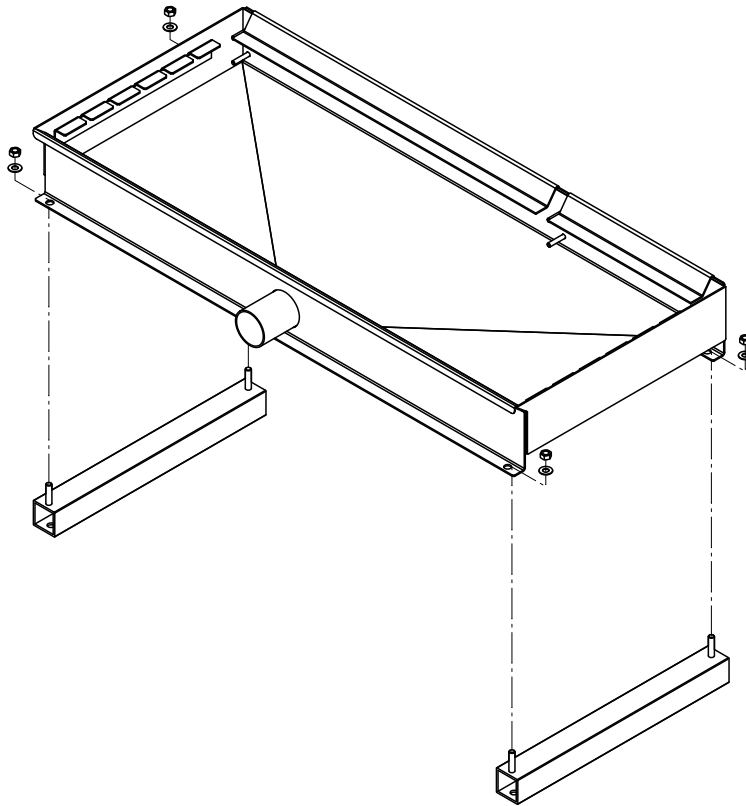
Abb. 5: Unterkonstruktionsprofile am Tank befestigen
