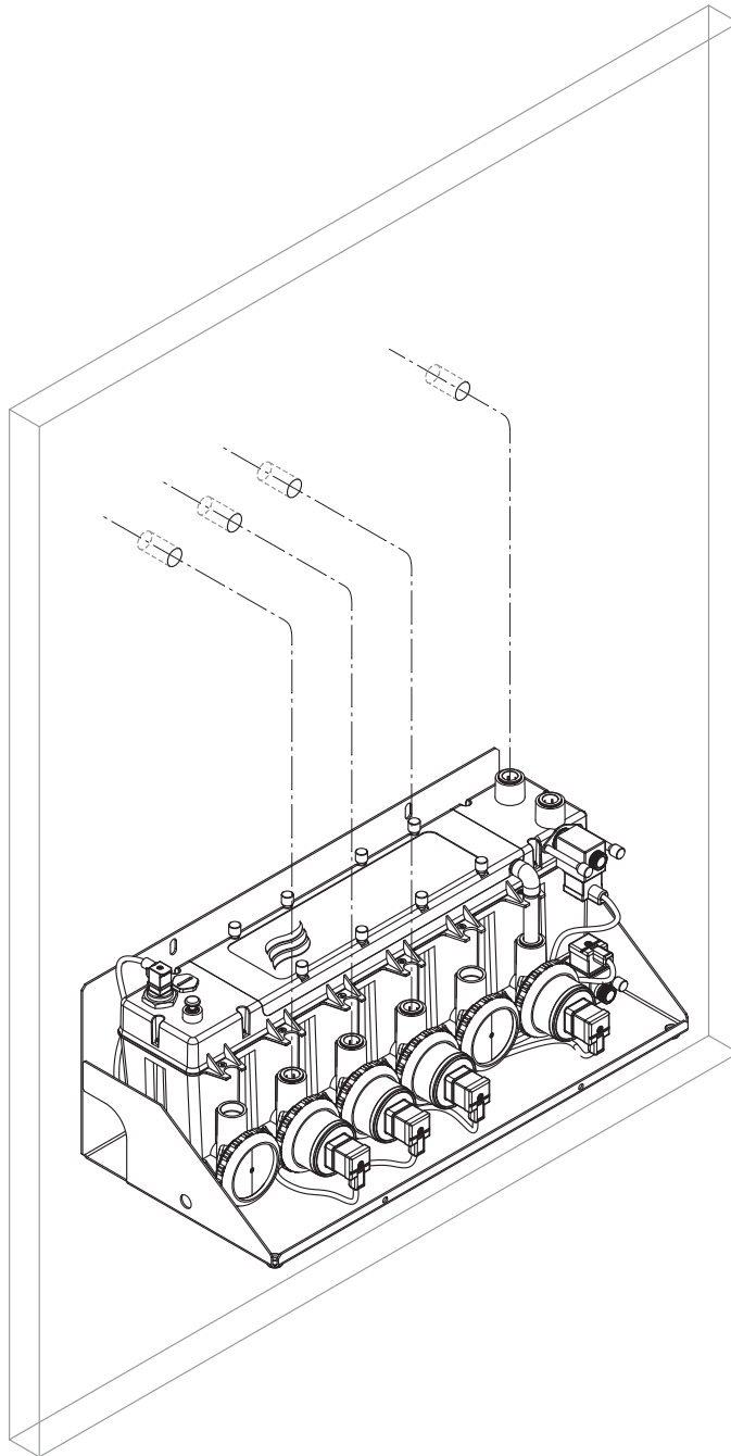
Abb. 24: Durchführungsbohrungen bohren (Aussenmontage)
