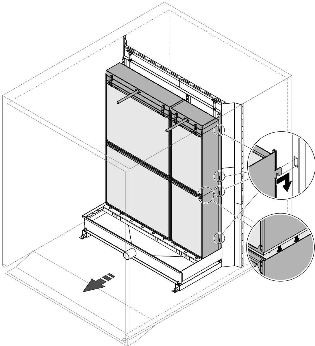
Abb. 14: Verdunsterkassetten montieren
