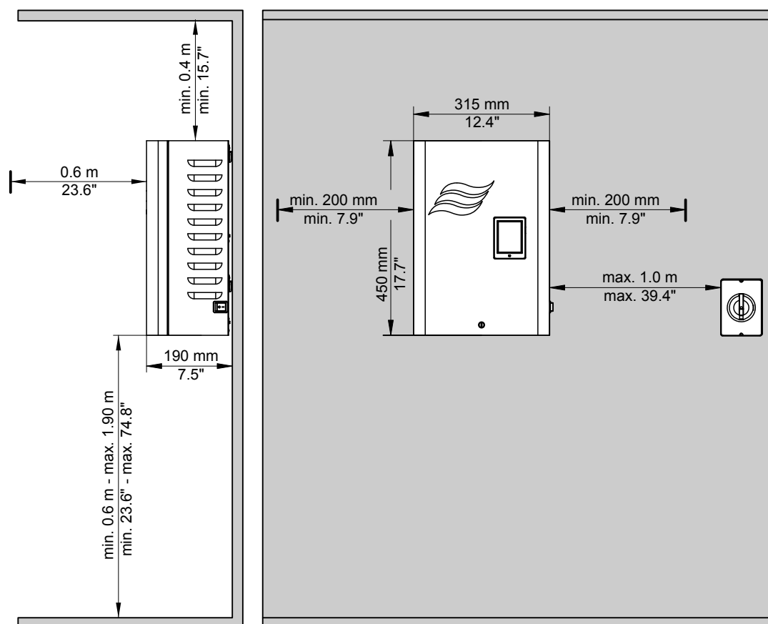
Abb. 32: Empfohlene Minimalabstände Steuereinheit
