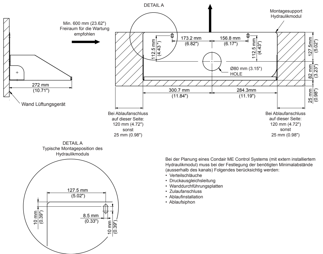
Abb. 19: Einzuhaltende Minimalabstände bei externer Montage des Hydraulikmoduls
