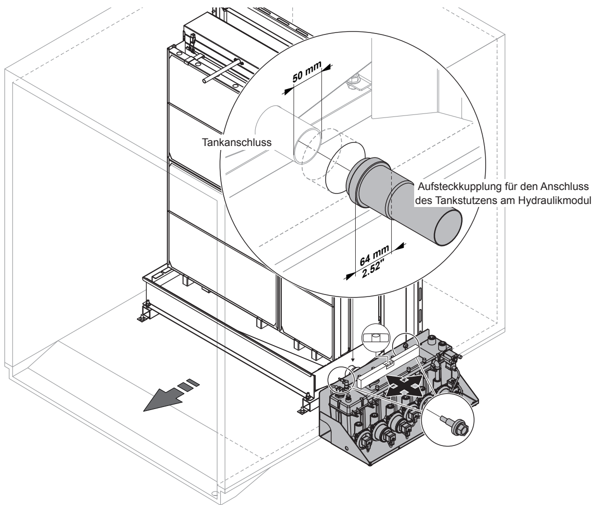
Abb. 21: Hydraulikmodul montieren (Aussenmontage, Wassertank mit Seitenablauf)
