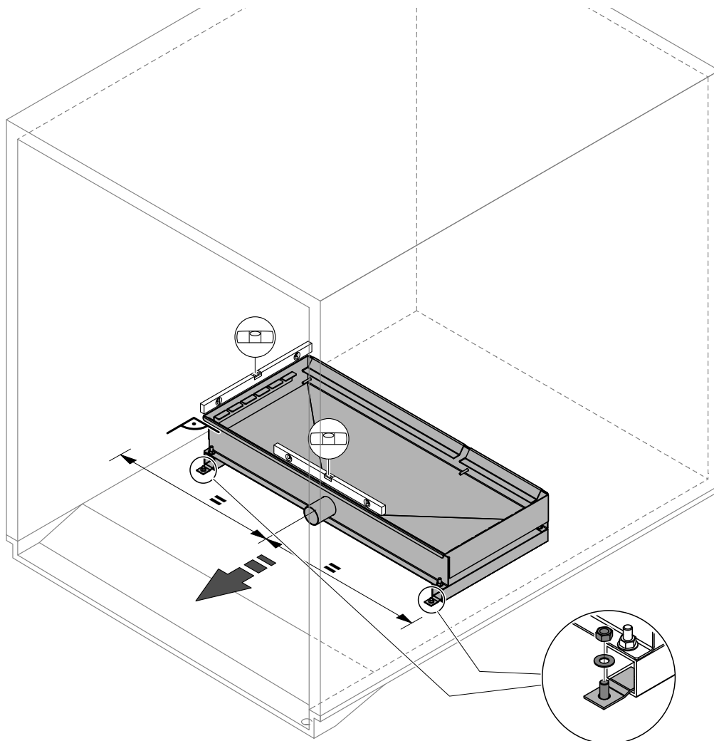
Abb. 6: Wassertank montieren
