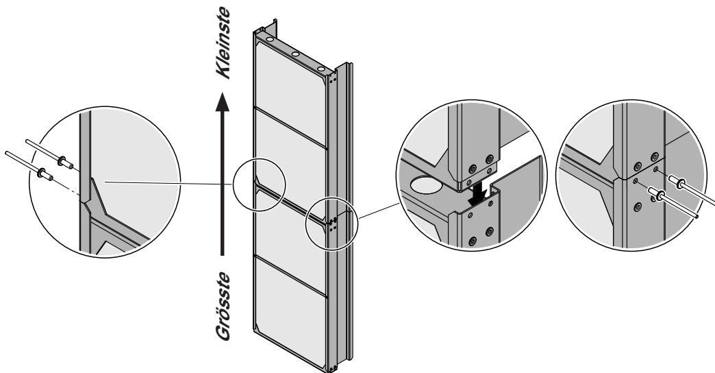
Abb. 16: Vertikalen Reihen der Tropfenabscheiderkassetten zusammennieten
