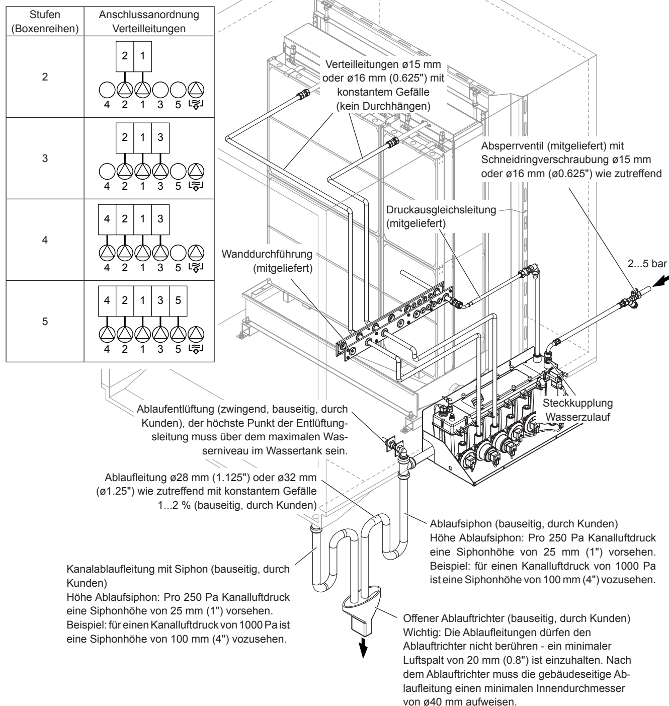
Abb. 31: Wasserinstallation (Aussenmontage)
