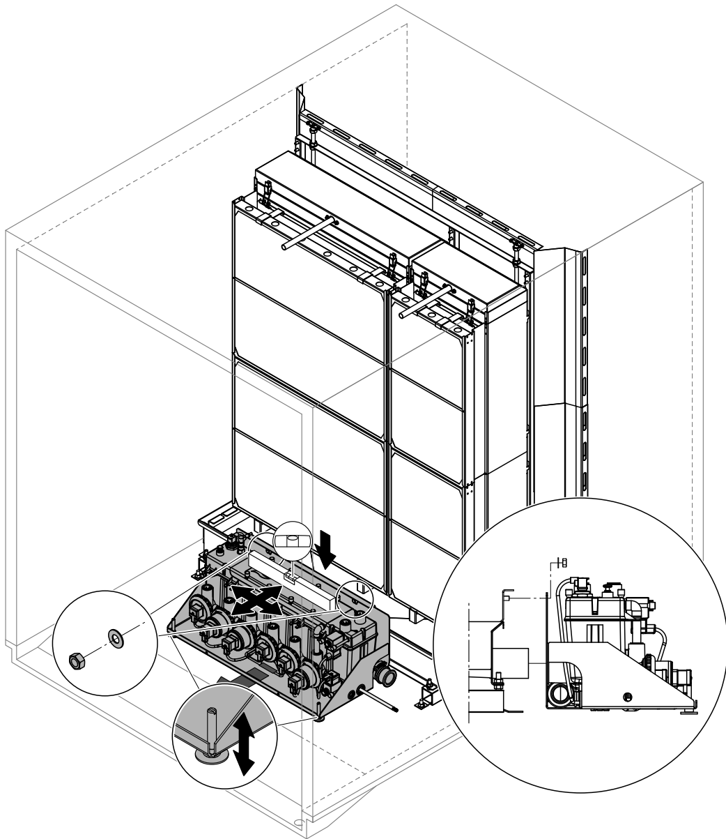
Abb. 18: Hydraulikmodul montieren (Innenmontage)
