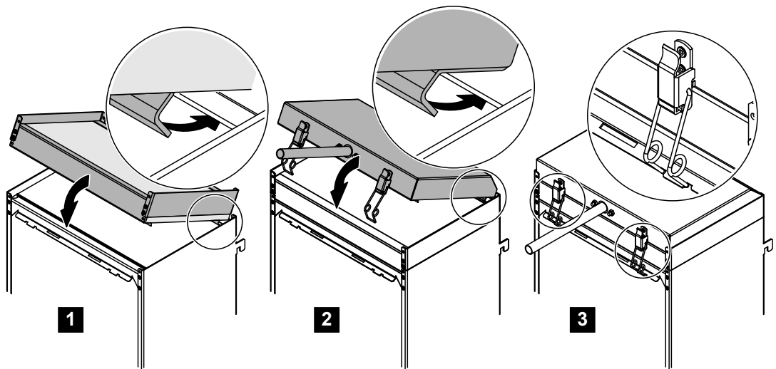
Abb. 12: Verteilhaubenzusammenbau auf der obersten Glasfaser-Verdunsterkassette montieren
