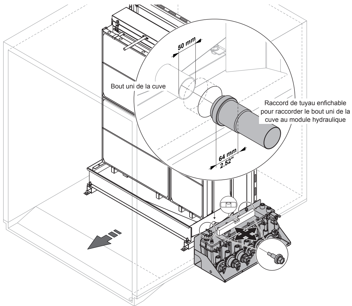
Fig. 21 : Montage du module hydraulique (installation externe, cuve de vidange latérale)
