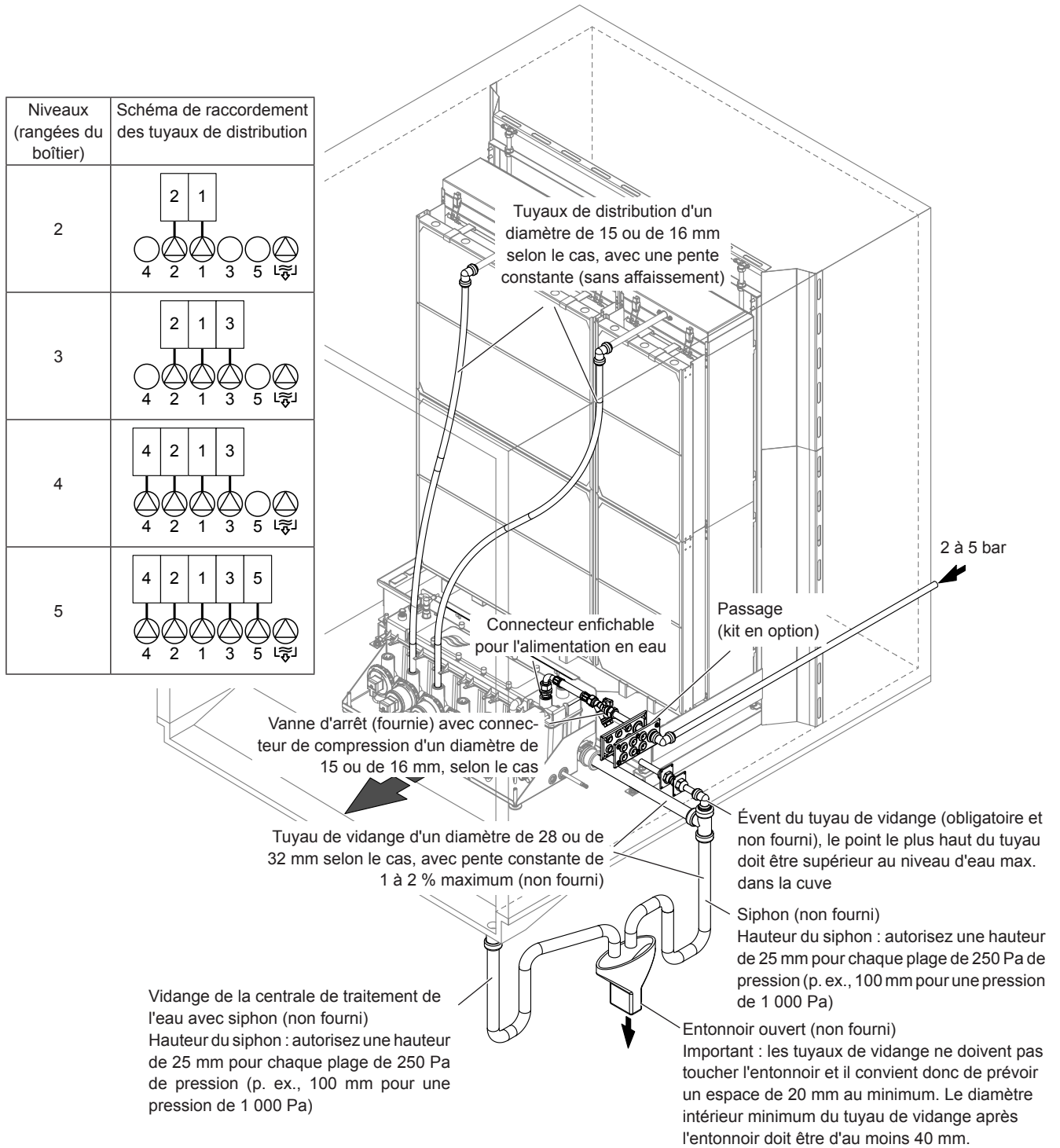
Fig. 30 : Installation du circuit d'eau (installation interne)
