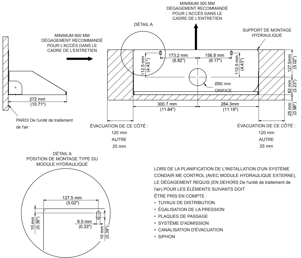
Fig. 19 : Espaces à respecter lors du montage externe du module hydraulique
