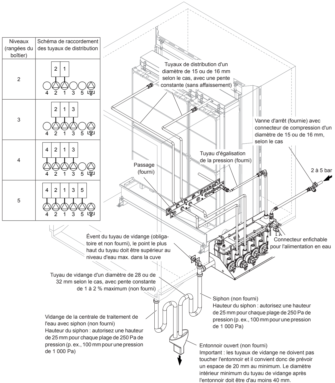
Fig. 31 : Installation du circuit d'eau (installation externe)
