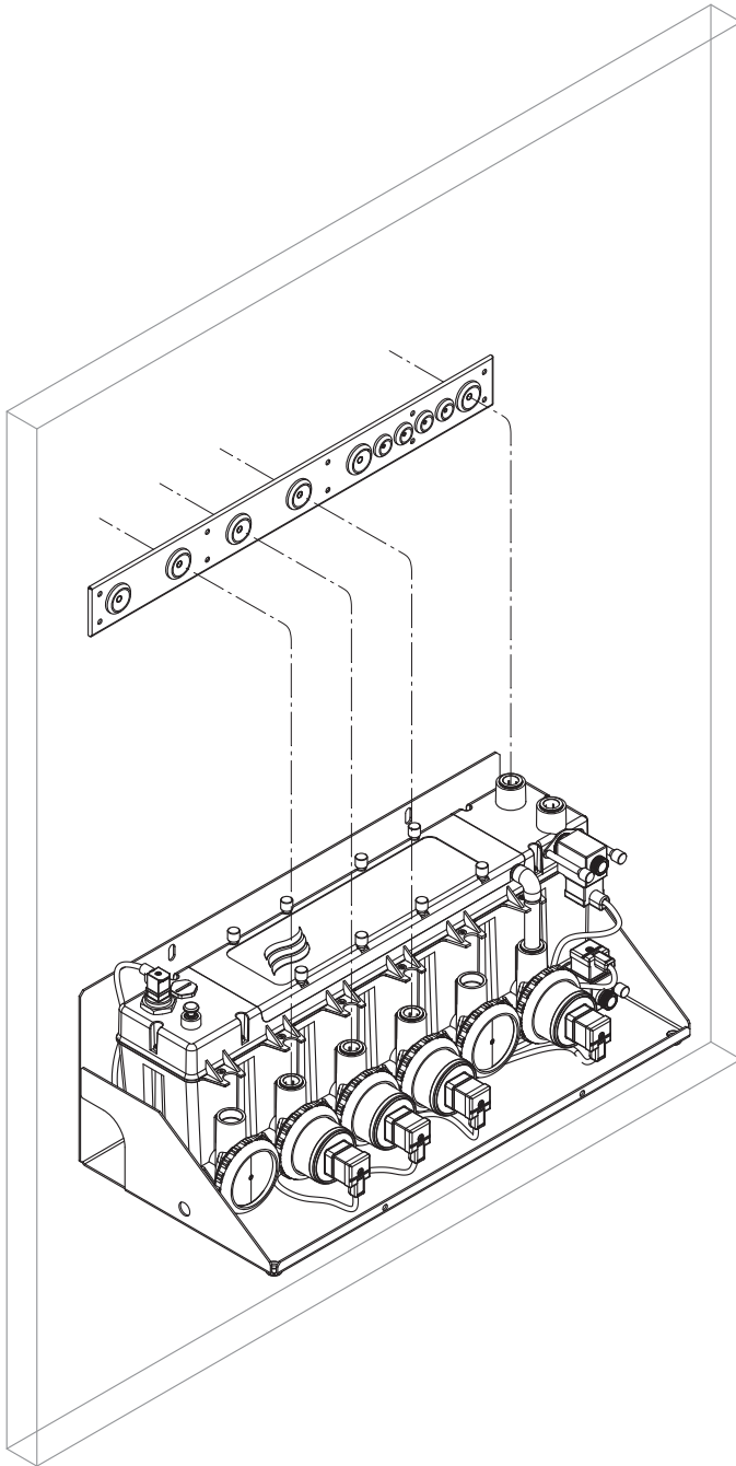
Fig. 22 : Marquage des orifices de passage (installation externe)
