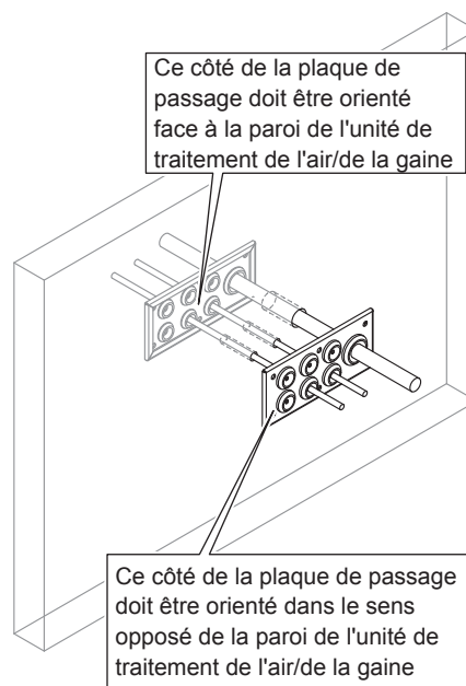
Fig. 27 : Montage de la plaque de passage (installation interne)
