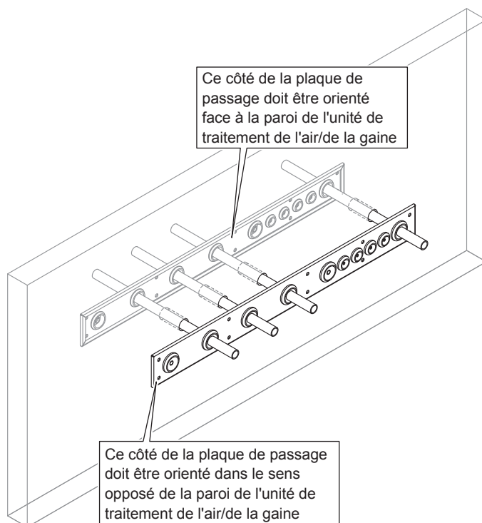
Fig. 26 : Montage de la plaque de passage (installation externe)
