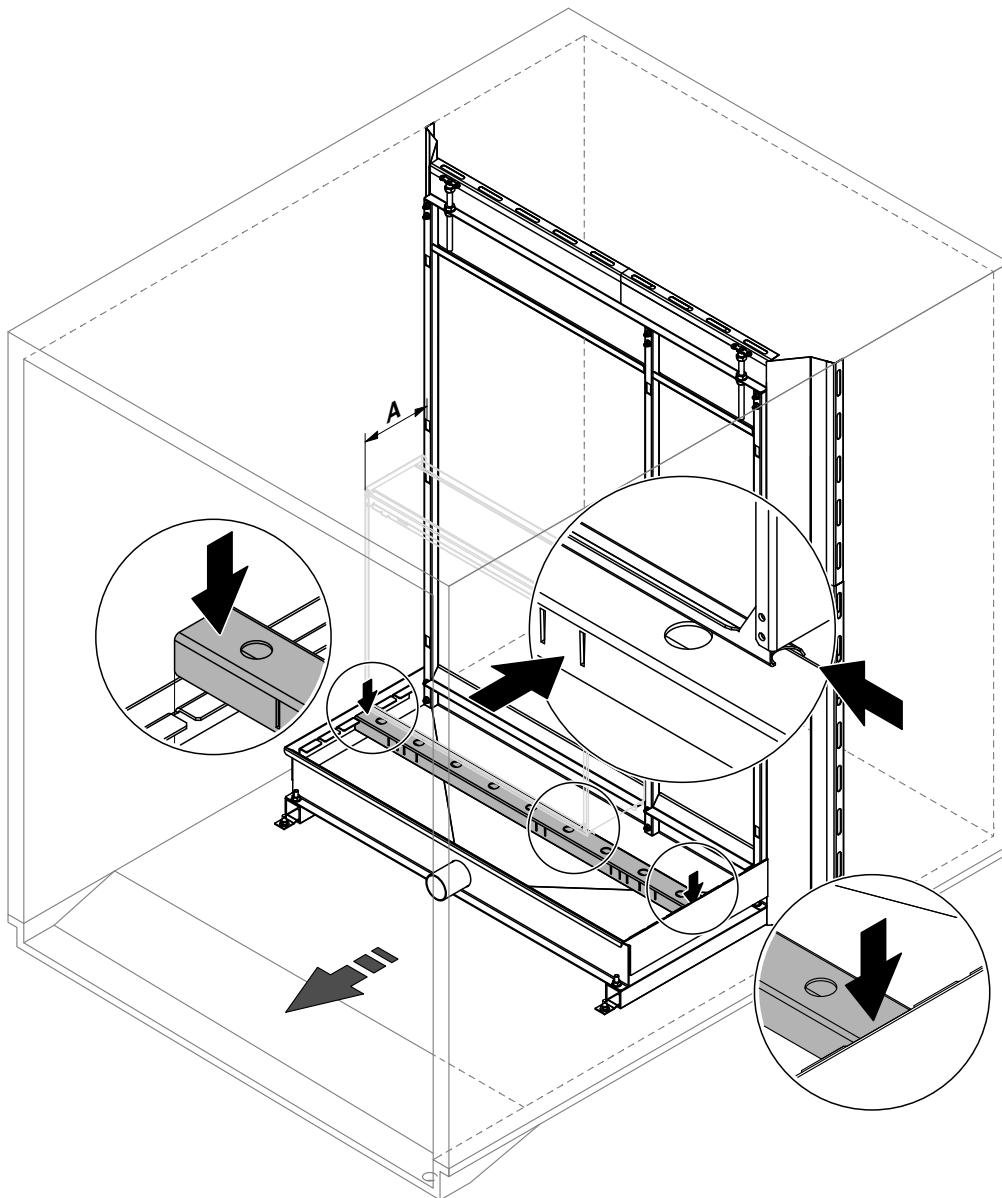
Fig. 11 : Montage de la barre transversale
