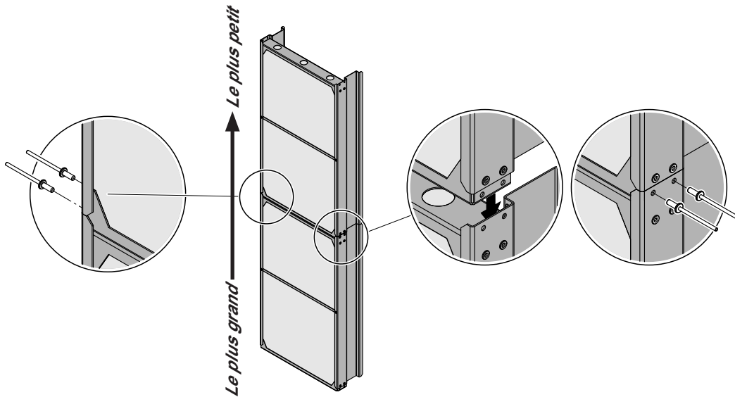
Fig. 16 : Rivetage des bancs des cassettes de séparateur de gouttelettes ensemble
