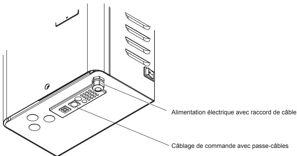
Fig. 34 : Passe-câbles de l'unité de commande
