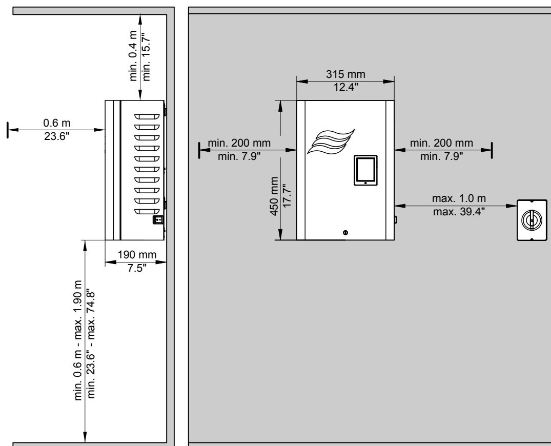
Fig. 32 : Recommandations en matière d'accessibilité de l'unité de commande
