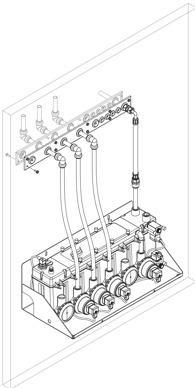
Fig. 28 : Fixation de la plaque de passage sur la paroi du conduit (installation externe)
