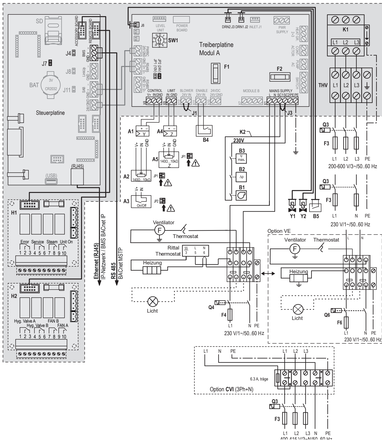
Bild 20: Anschlussschema für mittlere RS-Befeuchter
