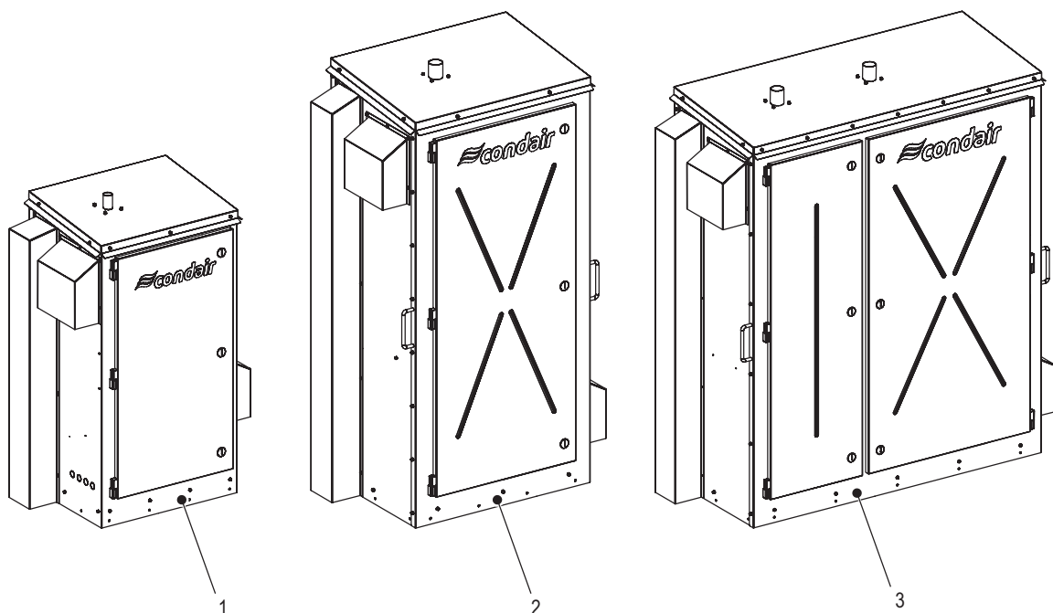
Bild 1: Condair EL/RS-Befeuchter – Gerätegrößen
