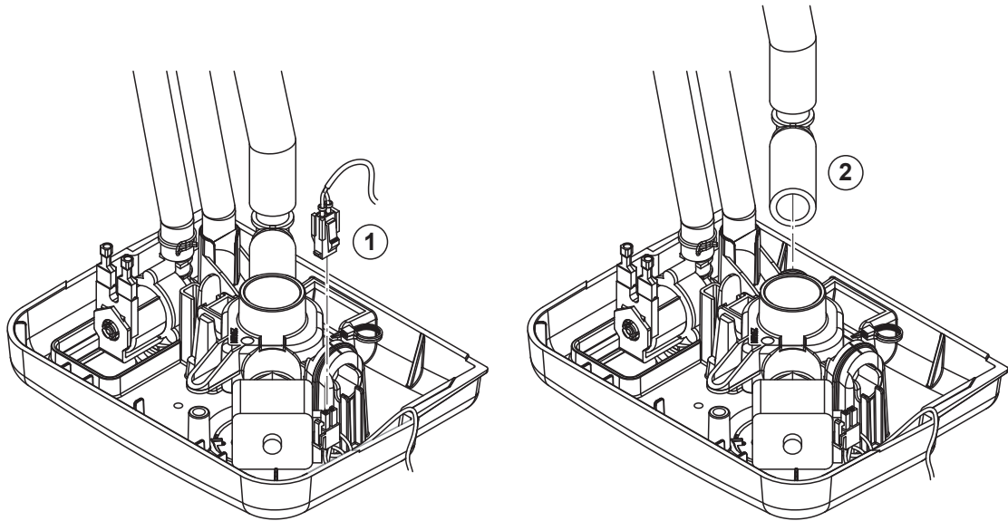
Abb. 10: Anschlusskabel ausstecken und Schlauch abziehen
