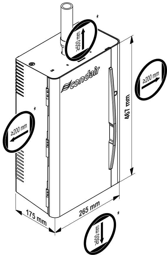
Abb. 5: Mindestabstände, Gerätedimensionen und Gewichte
