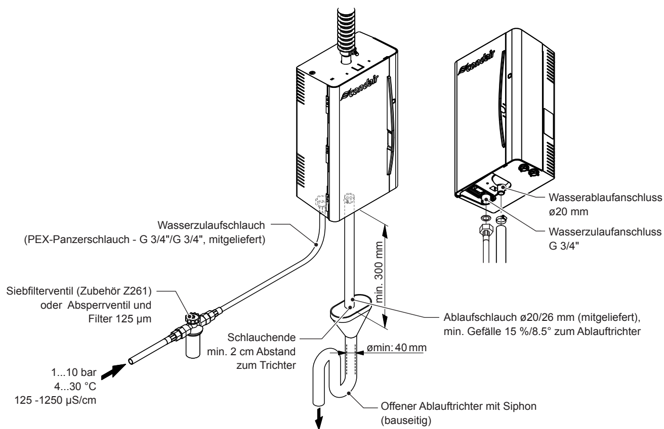
Abb. 7: Übersicht Wasserinstallation
