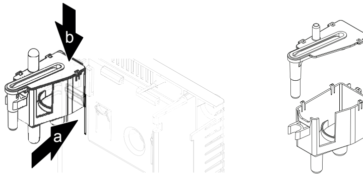
Abb. 15: Ausbau des Füllbechers und der Schläuche
