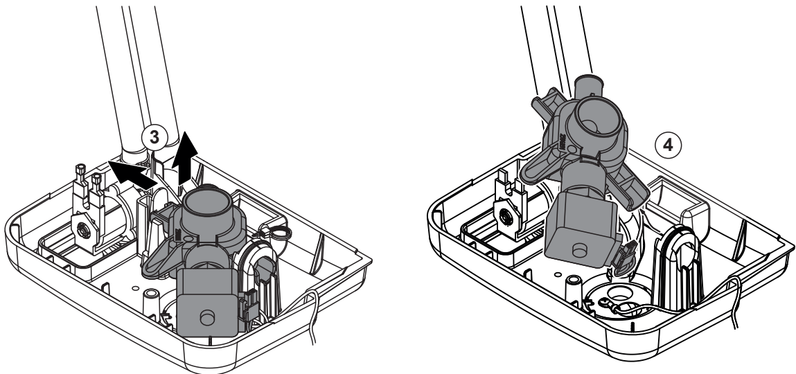
Abb. 11: Ausbau des Ablassventils
