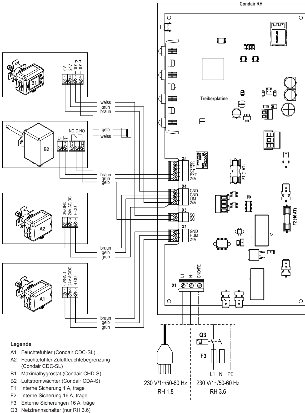
Abb. 8: Elektroschema Condair RH
