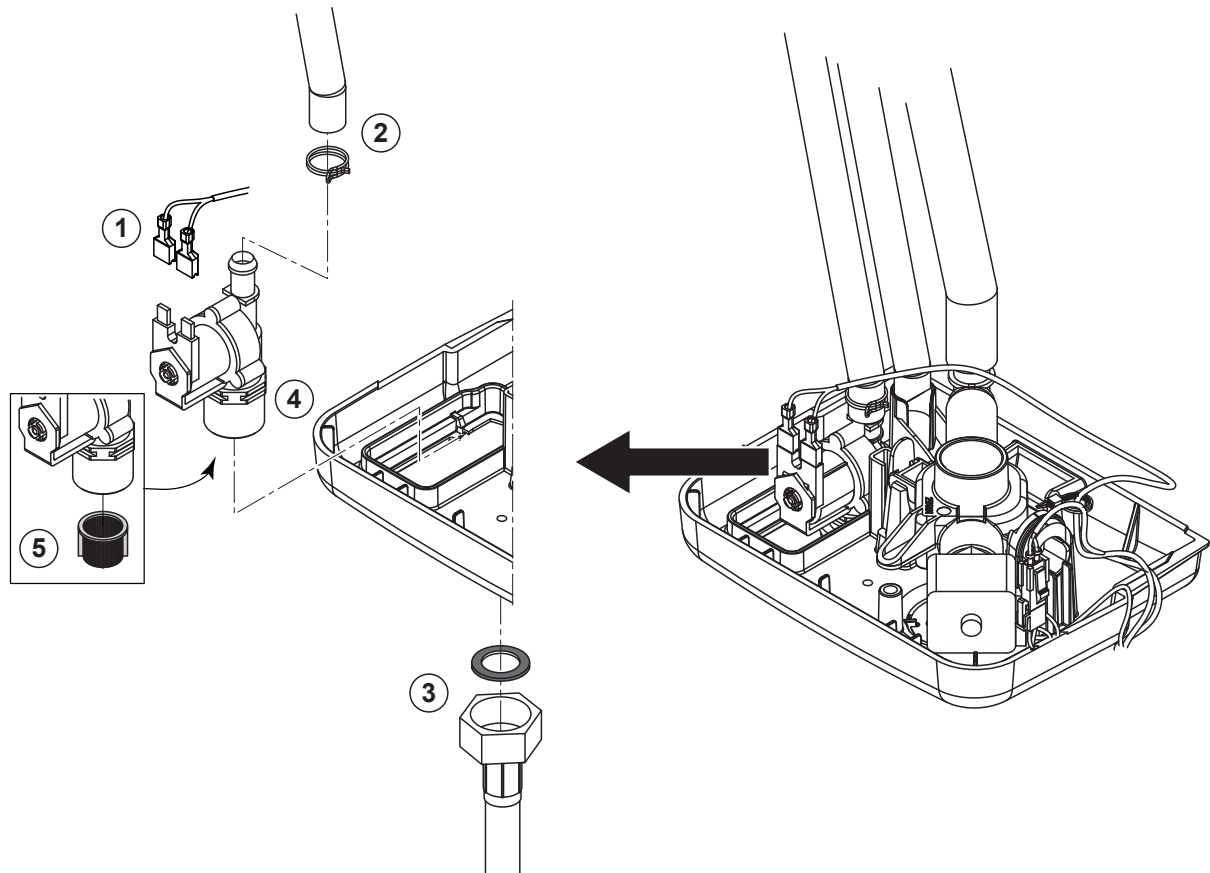
Abb. 14: Ausbau des Einlassventils
