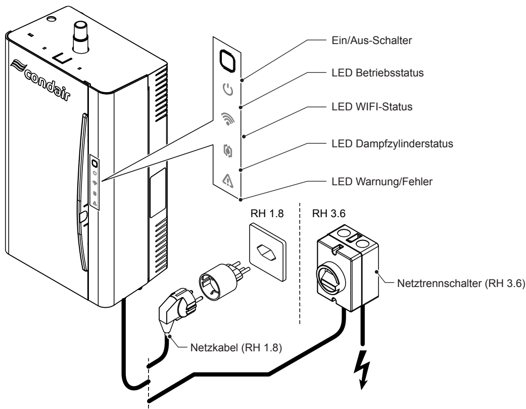
Abb. 9: Übersicht Anzeige- und Bedienelemente
