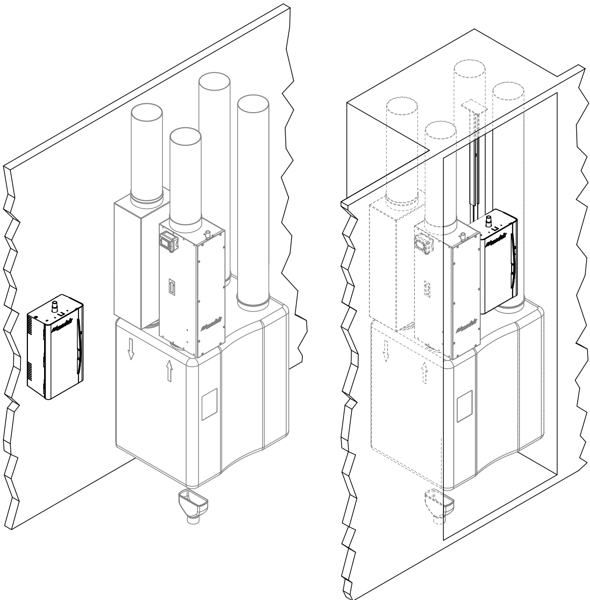
Abb. 6: Beispiel: Wand- und Deckenmontage Condair RH
