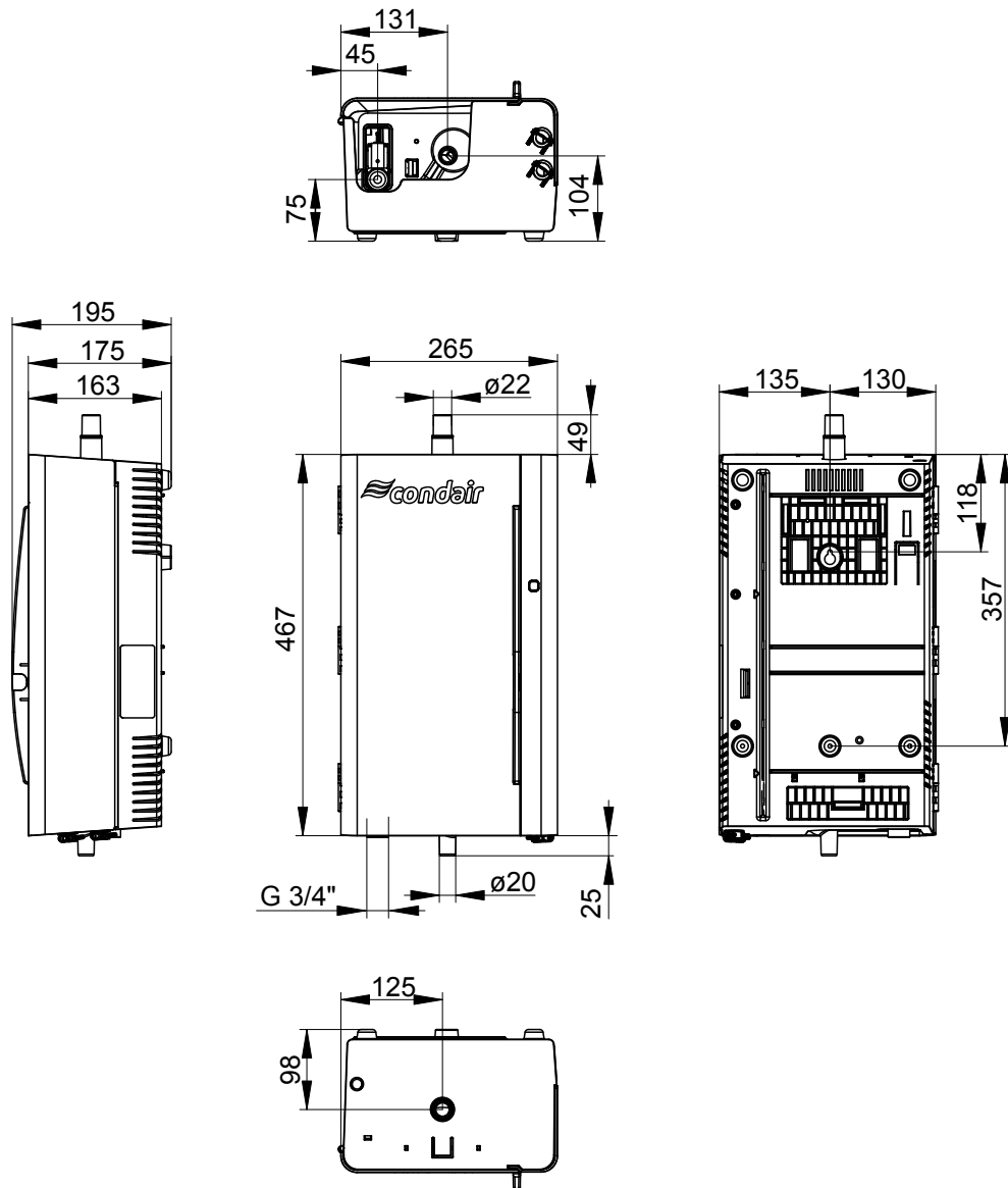
Abb. 16: Masszeichnung Condair RH (Masse in mm)
