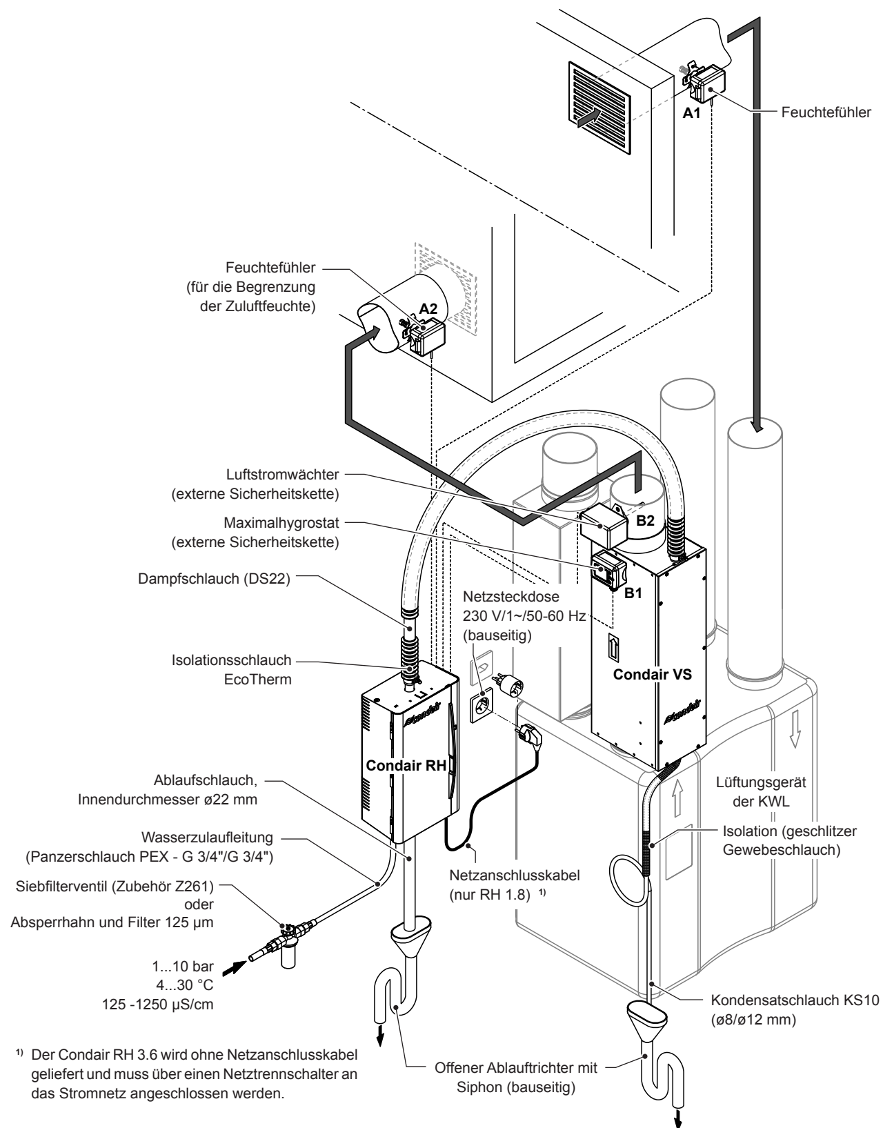
Abb. 2: Systemübersicht Condair RH mit Condair VS (Beispiel)
