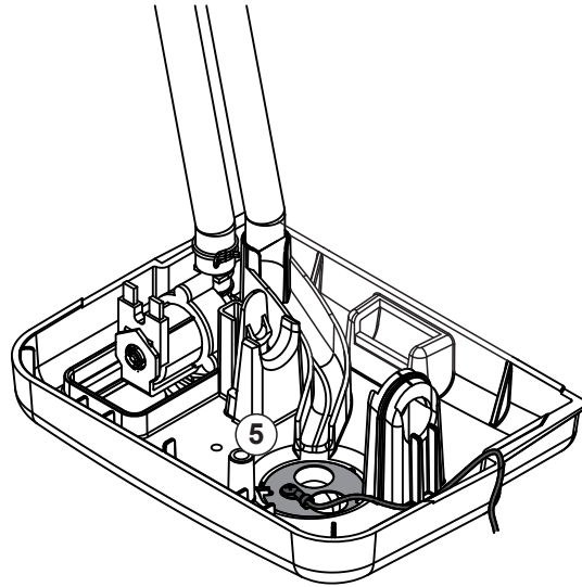
Abb. 12: FI-Schutzscheibe ausbauen
