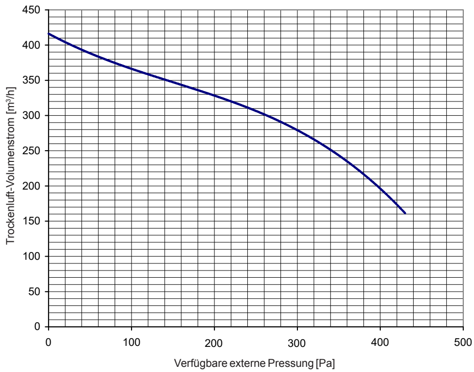
Abb. 20: Trockenluft-Volumenstrom Condair DA 400
