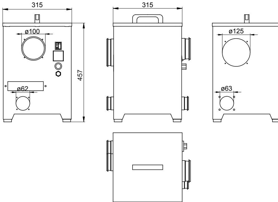
Abb. 14: Maßzeichnung Condair DA 210 (Masse in mm)
