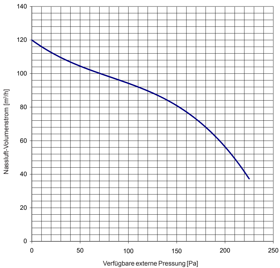
Abb. 24: Nassluft-Volumenstrom Condair DA 450
