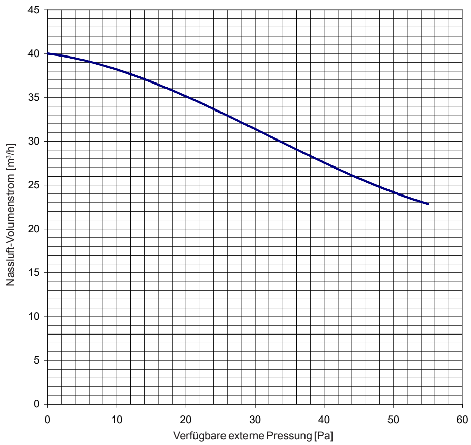
Abb. 18: Nassluft-Volumenstrom Condair DA 210
