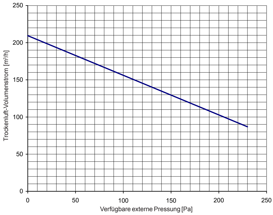
Abb. 17: Trockenluft-Volumenstrom Condair DA 210
