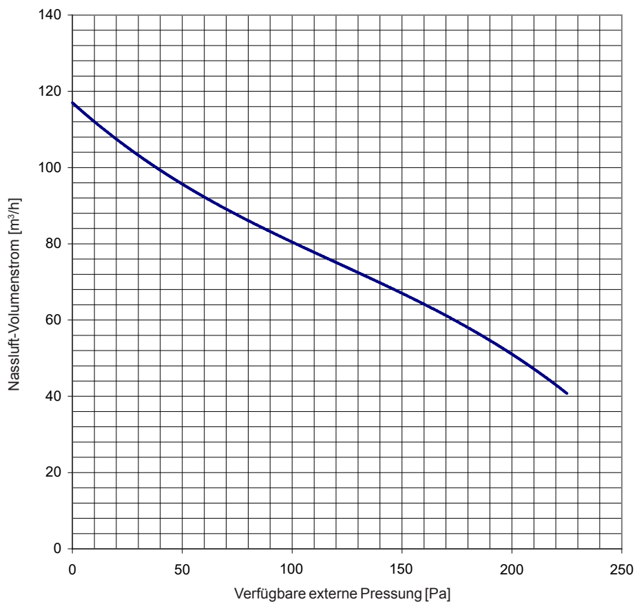
Abb. 21: Nassluft-Volumenstrom Condair DA 400
