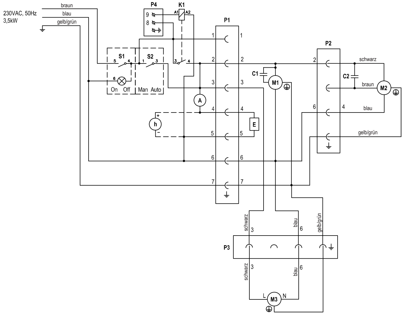
Abb. 26: Elektrischer Schaltplan Condair DA 400
