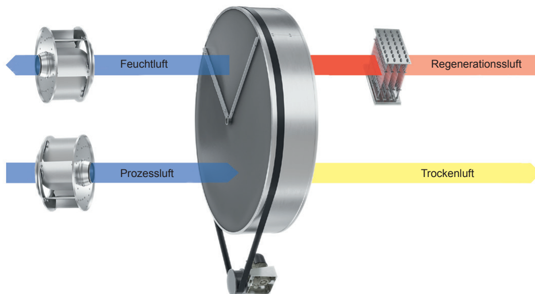
Abb. 2: Funktionsprinzip
