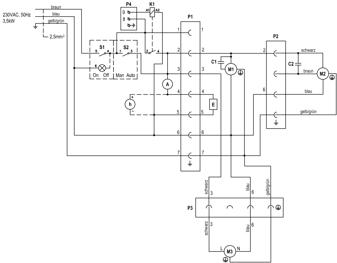
Abb. 27: Elektrischer Schaltplan Condair DA 450
