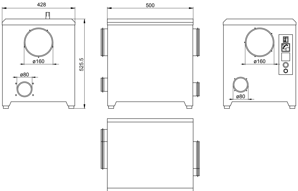
Abb. 15: Maßzeichnung Condair DA 400 - 450 (Masse in mm)
