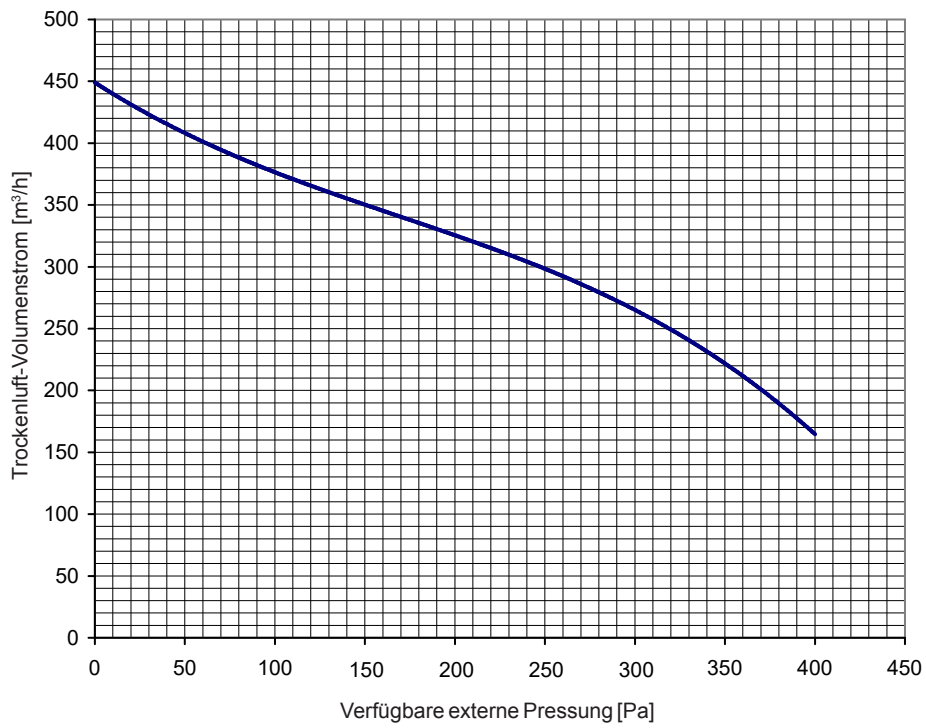
Abb. 23: Trockenluft-Volumenstrom Condair DA 450
