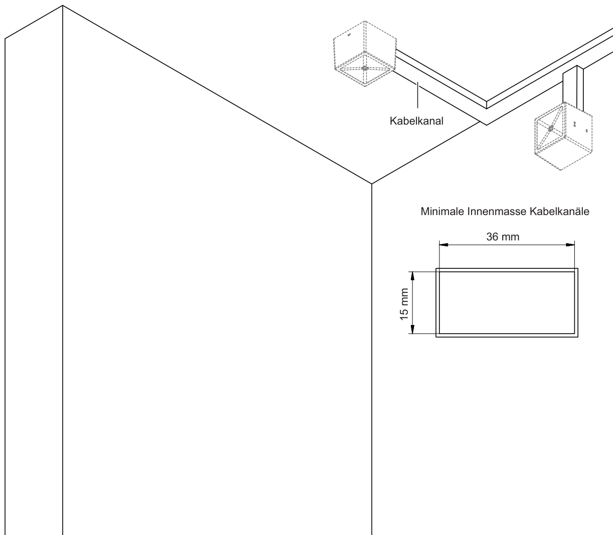
Abb. 23: Kabelkanäle verlegen
