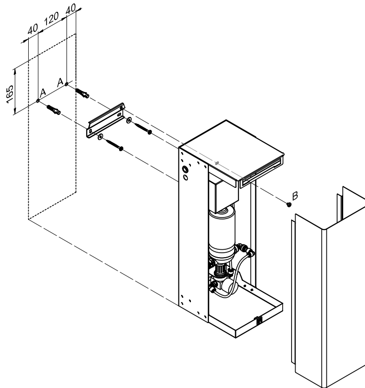
Abb. 25: Montage des Boostermoduls
